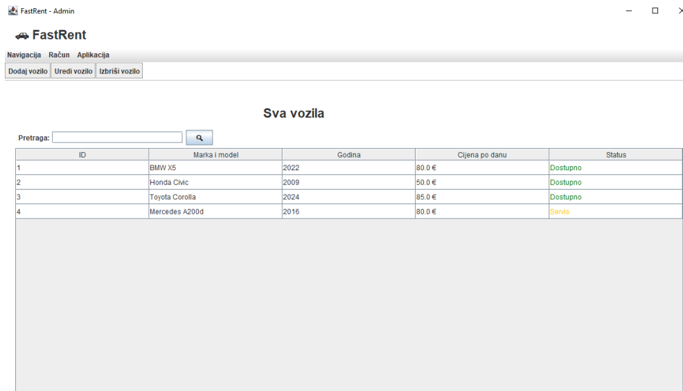
Slika 10: Sva vozila
