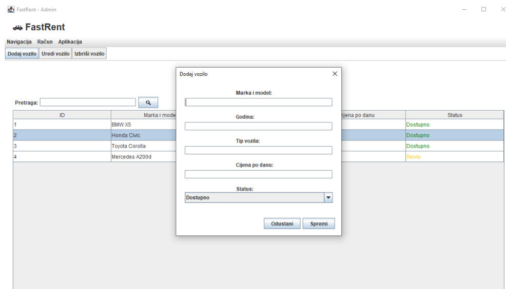
Slika 11: Dodaj vozilo
