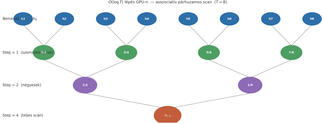
3.2. ábra. A Blelloch-féle párhuzamos prefix-scan vizualizációja 8 elemű szekvencián. Minden lépésben a step -nyi távolságú két elem kombinálódik; \log_2 T = 3 lépés után minden h_t tartalmazza az előzmény-összesítést. Ez teszi lehetővé a szekvenciális állapotfrissítés hatékony GPU-s párhuzamosítását.
