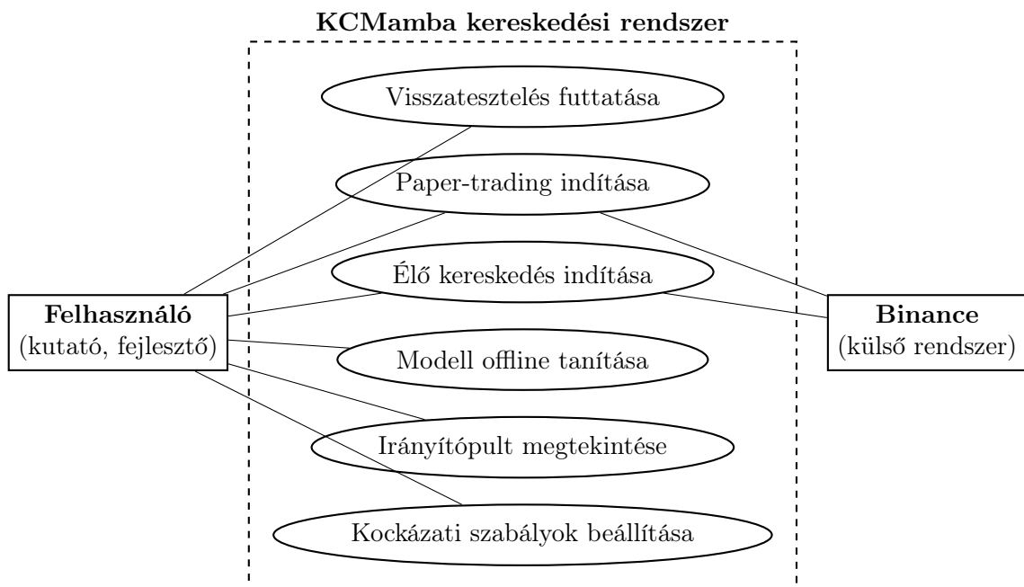
5.6. ábra. A KCMamba rendszer használati esetei. A felhasználó hat fő művelethez fér hozzá; a Binance külső rendszerként a paper- és élő-kereskedési útvonalon kapcsolódik be (piaci adat, megbízás-végrehajtás).
