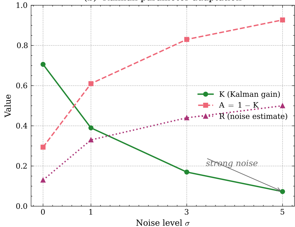
(b) Kalman parameter adaptation
