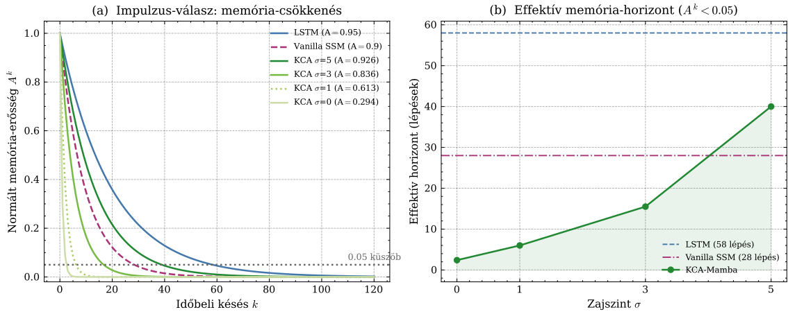
3.5. ábra. Bal: Impulzus-válasz függvény: az állapot exponenciális csökkenése h_k = A^k a késő k függvényében. A KCMamba A -értéke adaptívan nő a zajszinttel ( 0.294 \rightarrow 0.926 ), ezzel a memória-horizont is növekszik. Jobb: Effektív memória-horizont (az a lépésszám, ameddig A^k > 5\% ) a zajszint függvényében. Az LSTM és vanilla SSM rögzített horizonttal rendelkeznek, a KCMamba zajban automatikusan hosszabb memóriát tart fenn.
