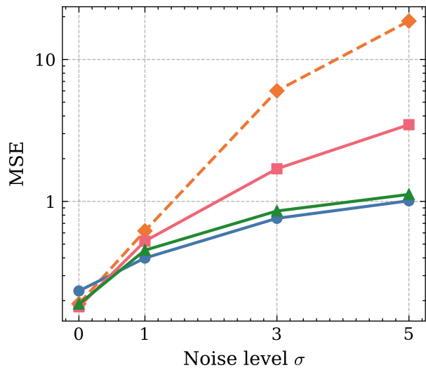
ETTh1, s = 16
