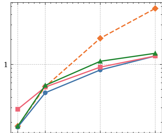
ETTh2, s = 16
