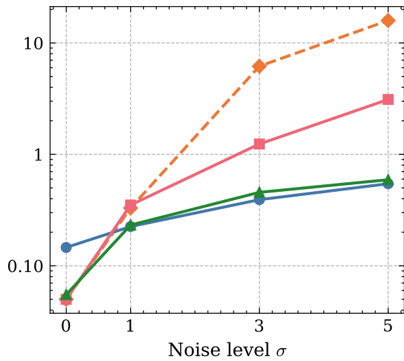
ETTh2, s = 16
