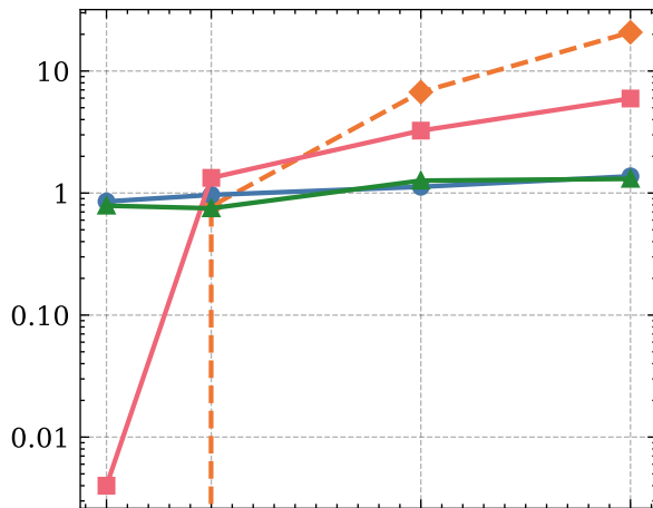
ETTh2, s = 1
