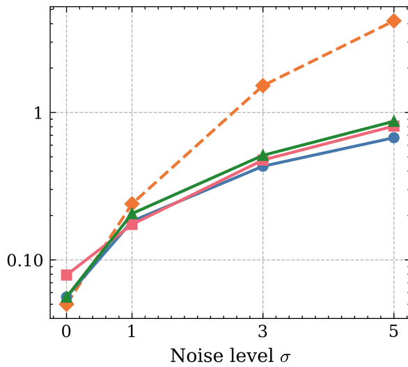
ETTh2, s = 1
