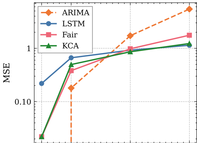
ETTh1, s = 16
