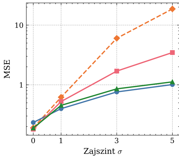
ETTh1, s = 16
