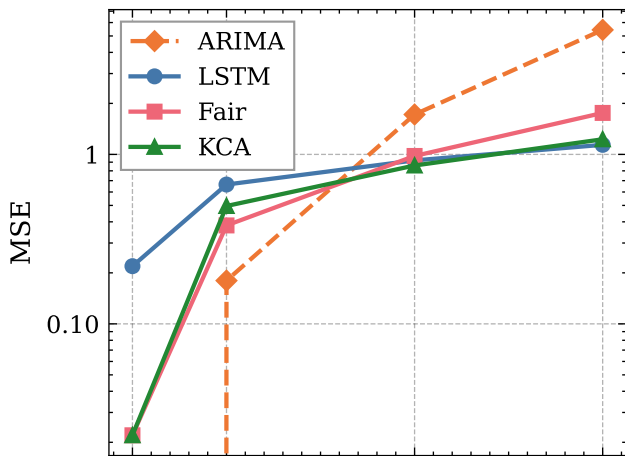
ETTh1, s = 16
