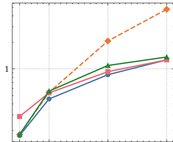
ETTh2, s = 16
