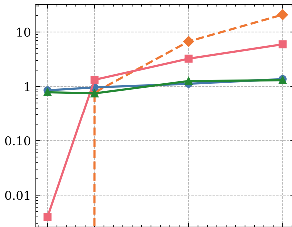
ETTh2, s = 1
