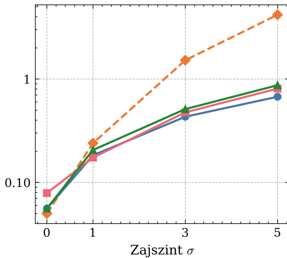
ETTh2, s = 1
