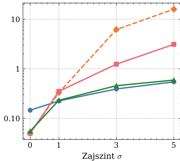
ETTh2, s = 16
