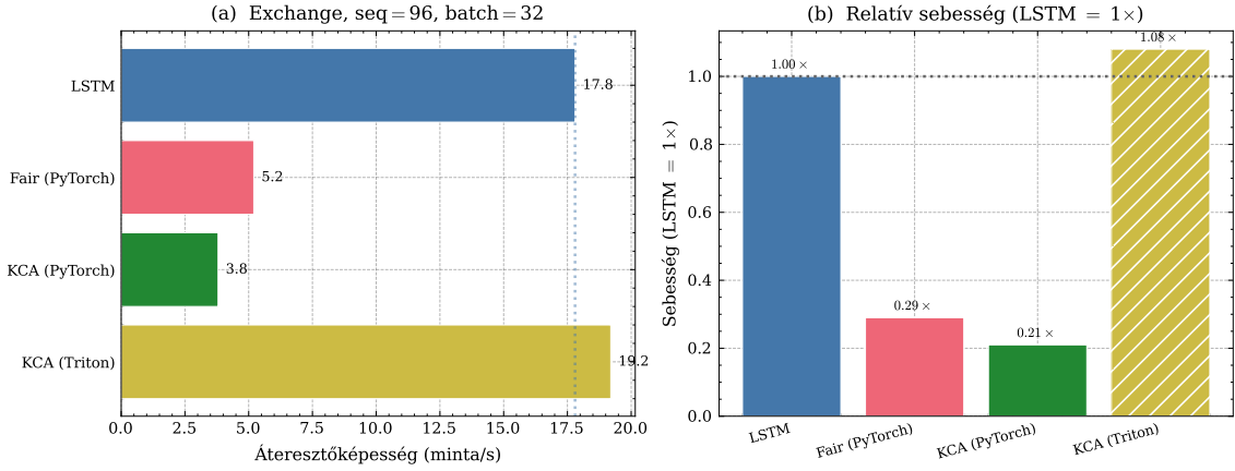
4.7. ábra. Bal: Áteresztőképesség (minta/s) T = 96 -nál, kötegméret= 32, RTX 3060-on. A cuDNN-optimalizált LSTM a referencia; a naív PyTorch szelektív scan 3,4\times lassabb, egy Triton-kernelre írt KCMamba viszont LSTM-szintű sebességet ér el. Jobb: LSTM-hez normált relatív sebesség. A Triton-kernel rövid szekvenciákon szükséges, de nem elégséges optimalizáció. T \geq 2000 -nél a scan O(\log T) mélysége várhatóan 2\text{--}10\times -es előnyt ad a szelektív SSM-ek irodalmában [2].
