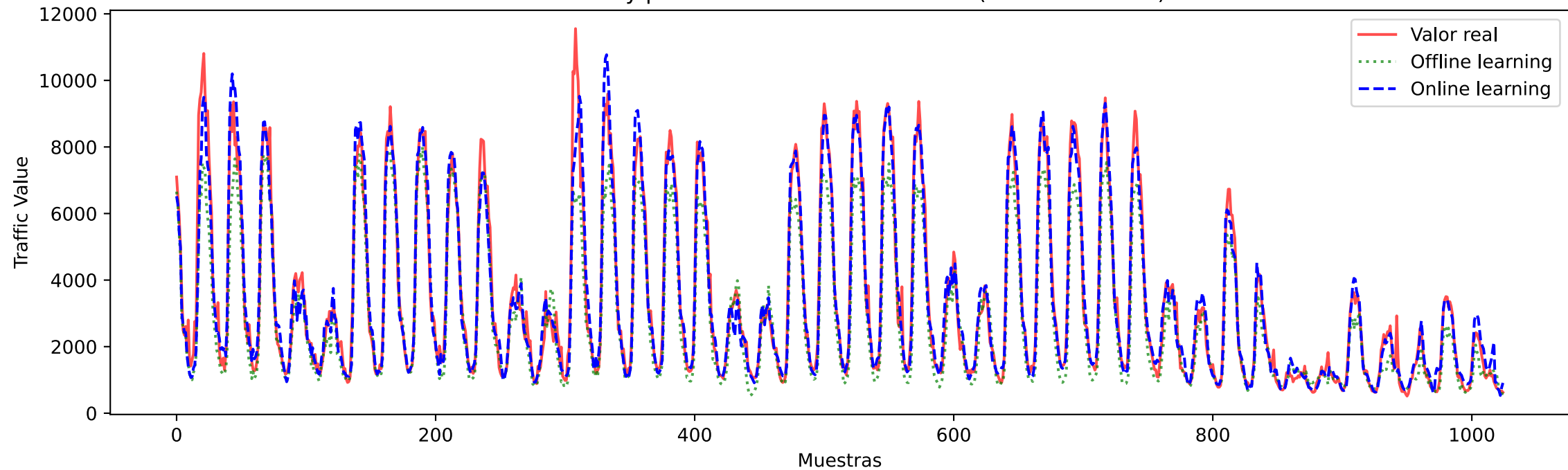
Valor real y predicción de la celda #5063 (RNMSE: 0.1953)
