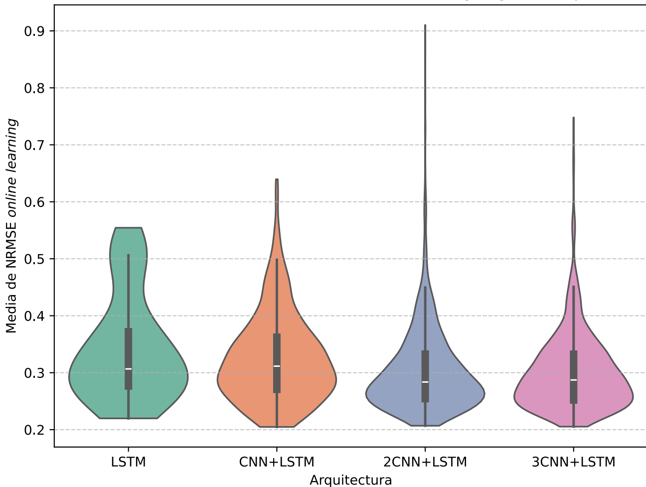
Distribución de las medias de NRMSE online learning según la arquitectura
