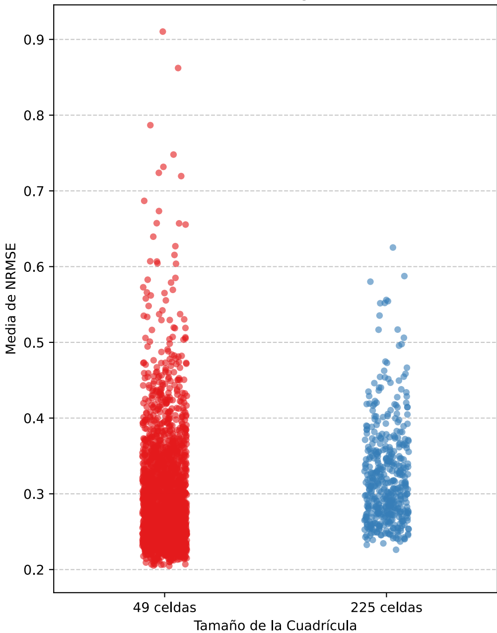
Distribución de las medias NRMSE según el tamaño de la cuadrícula
