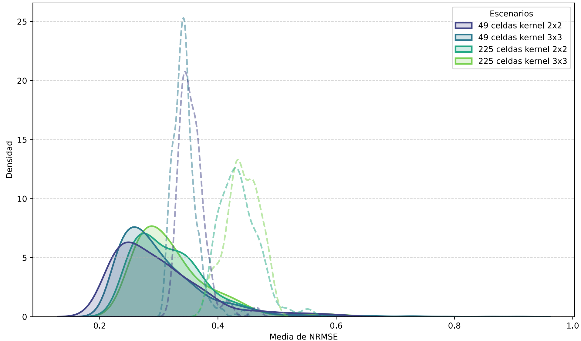
Densidad de las medias de NRMSE en entrenamiento estático (discontinua) y online learning (continua) según el tamaño de la cuadrícula y del kernel
