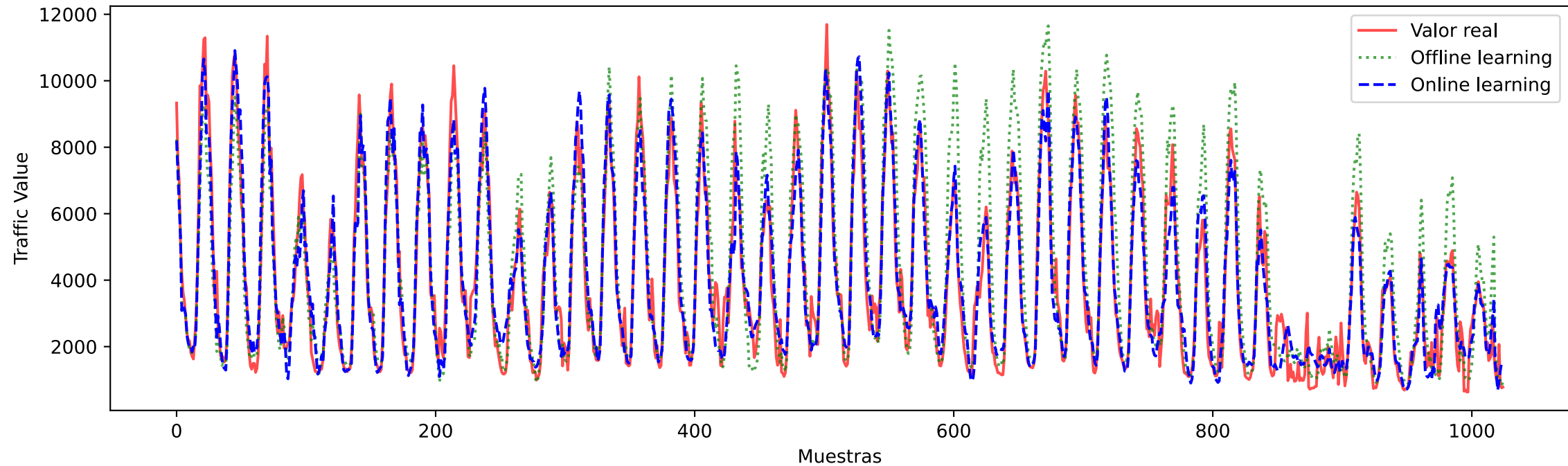
Valor real y predicción de la celda #4959 (RNMSE: 0.2852)
