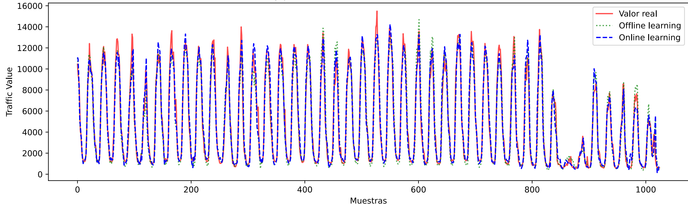
Valor real y predicción de la celda #5162 (RNMSE: 0.1778)
