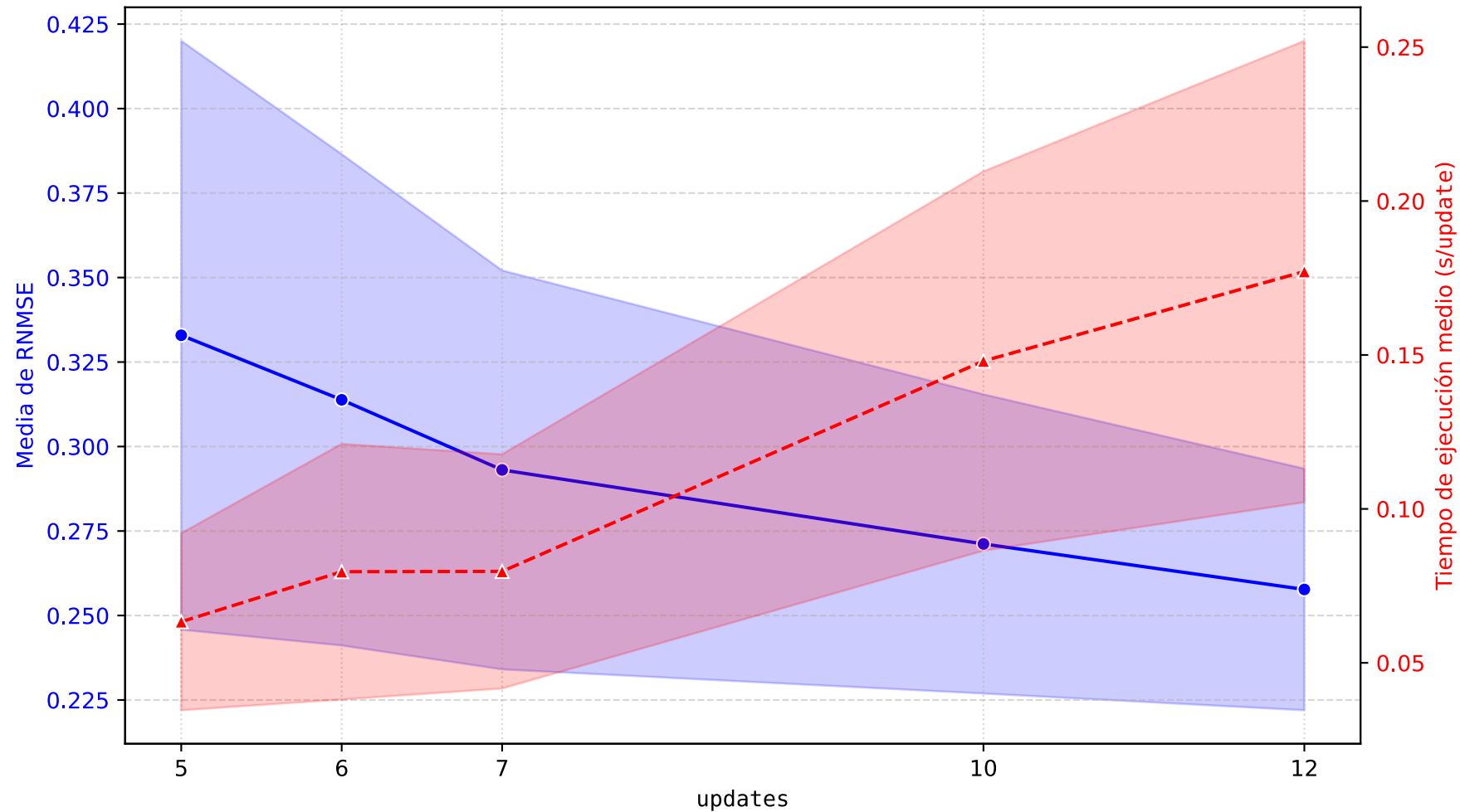
Impacto de updates en la media de NRMSE onlinelearning y del tiempo de ejecución
