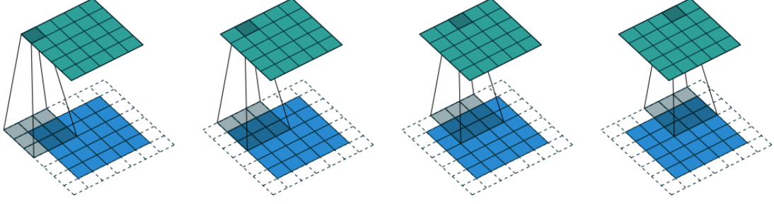
Figura 14: Ejemplo de capa convolucional 5x5 con entradas 5x5 con un perímetro de zero padding [55].
