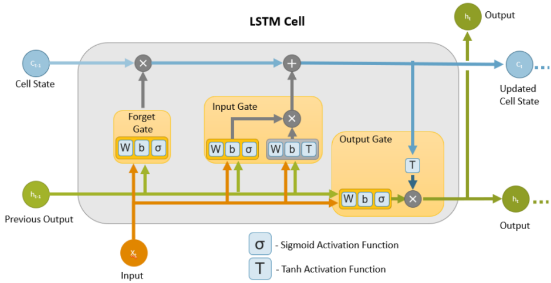
Figura 13: Representación de una neurona LSTM con todas sus elementos, puertas y operaciones [50].
