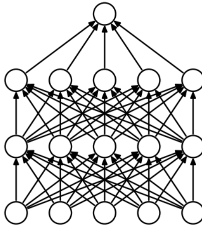
Figura 5: Estructura de un MLP [28].
