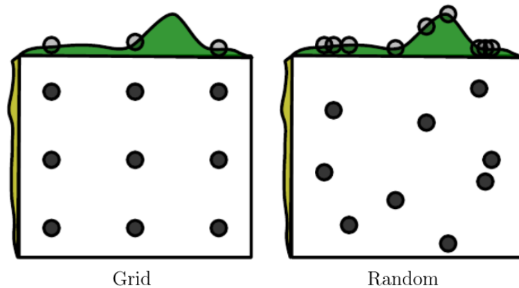
Figura 8: Comparación entre grid search y random search [22].
