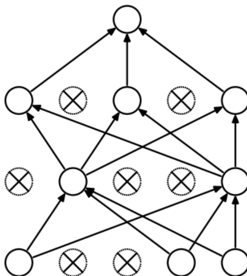
Figura 10: Ejemplo de un MLP con dropout durante el entrenamiento [28].
