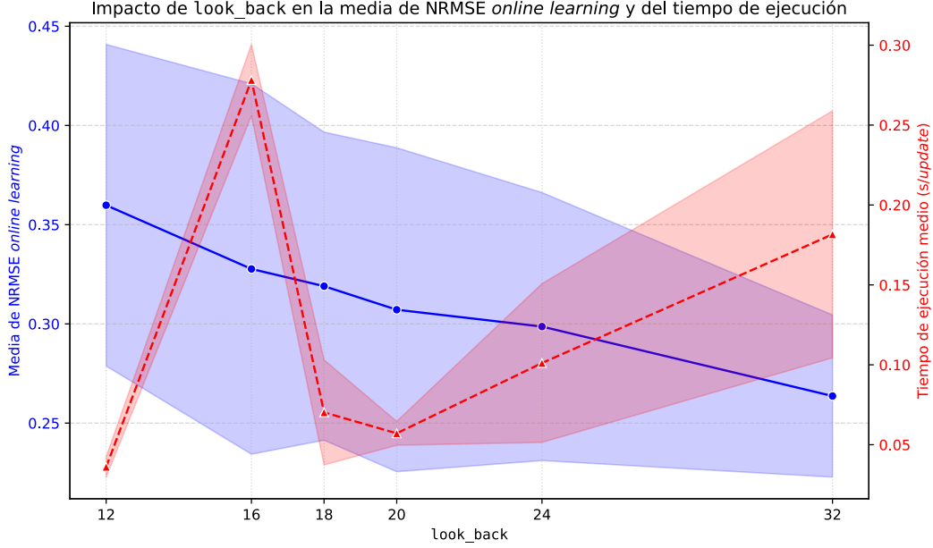
Figura 23: Influencia del hiperparámetro look_back en la media del NRMSE y en el tiempo de ejecución medio en modelos con online learning . Elaboración propia.
