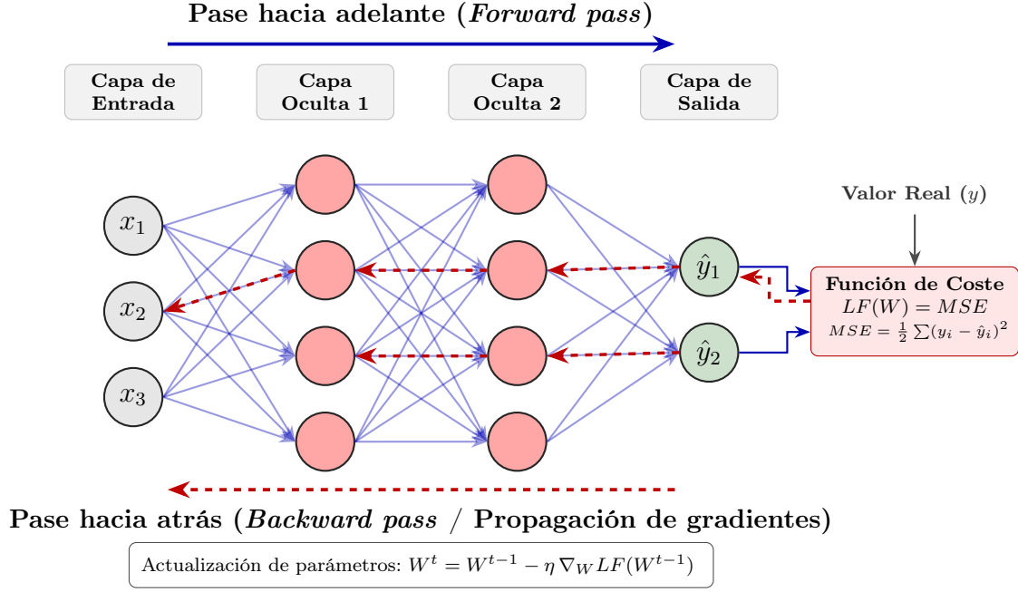
Figura 7: Ilustración del mecanismo de retropropagación. Elaboración propia
