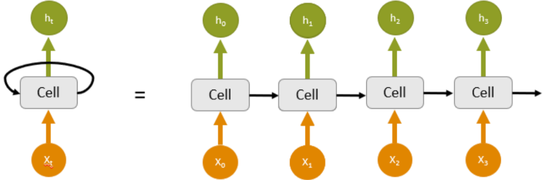
Figura 12: Representación de una neurona recurrente y su desglose en el tiempo [50]
