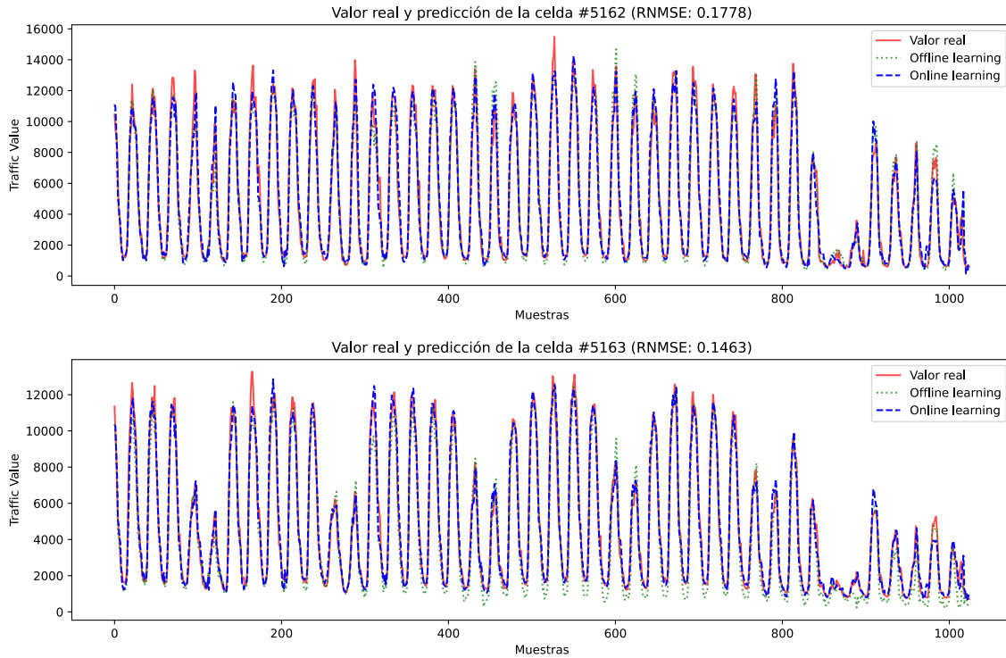
Figura 27: Tráfico real y predicciones con online y offline learning del mejor modelo en las celdas 5162 (arriba) y 5163 (abajo). Elaboración propia.
