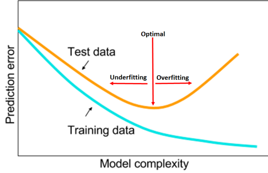
Figura 9: Gráfico explicativo de la relación entre el error de entrenamiento ( E_{in} ) y el error de test E_{out} [35]
