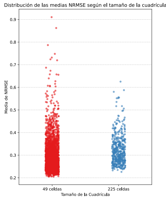
Figura 20: Distribución de las medias de NRMSE de los modelos con online learning según el tamaño de la cuadrícula. Elaboración propia.
