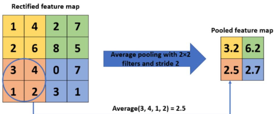
Figura 15: Ejemplo de capa pooling basada en la media aritmética de las celdas del campo visual con kernel 2x2 y stride 2 [57].
