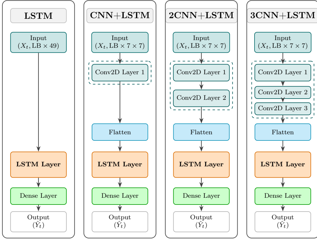
Figura 19: Comparación de las arquitecturas evaluadas: LSTM base, CNN+LSTM, 2CNN+LSTM y 3CNN+LSTM para una cuadrícula de 49 celdas. Elaboración propia.
