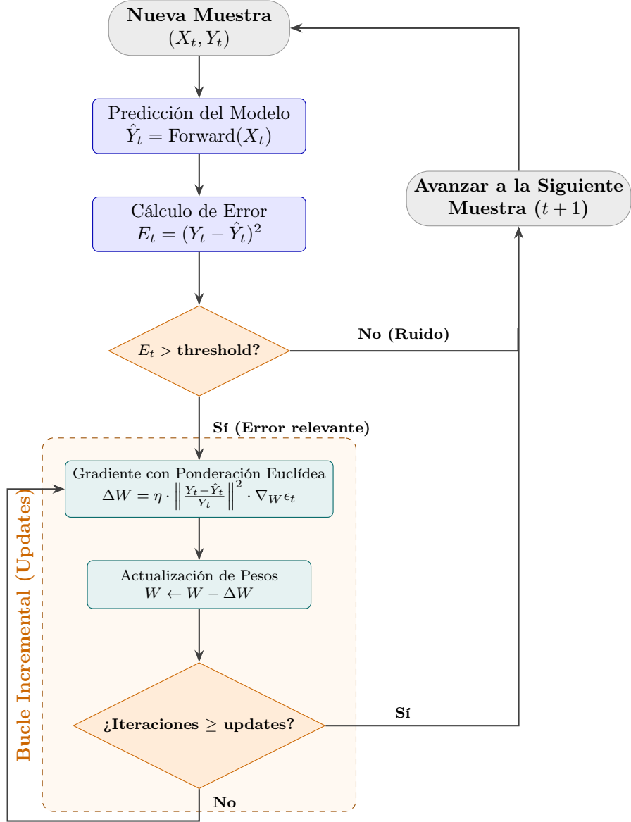
Figura 3: Diagrama de flujo del algoritmo de reentrenamiento online incremental con filtrado por umbral (threshold) y bucle de iteraciones (updates).
