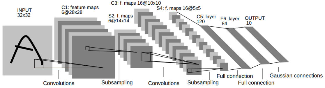
Figura 16: Ejemplo de una arquitectura CNN con capas convolucionales y de agregación intercaladas [56]
