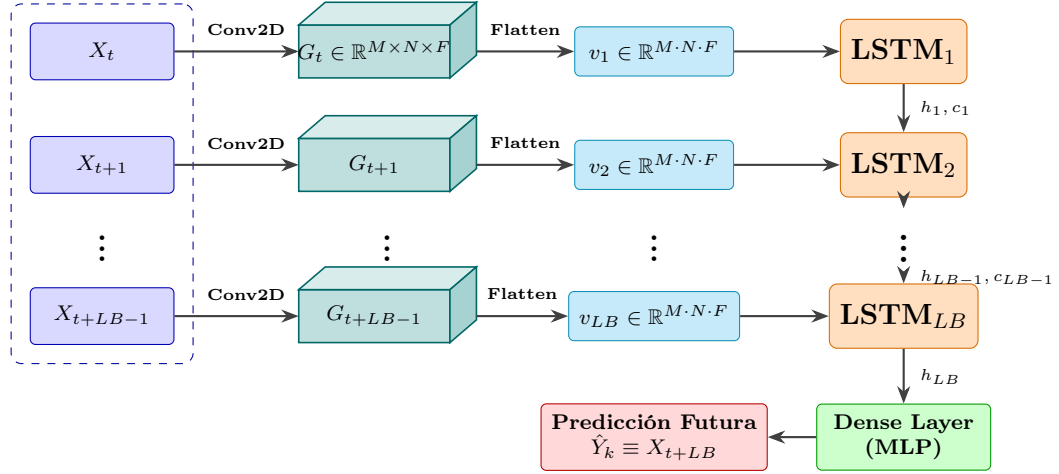
Figura 17: Ilustración del procesado de un mini-batch de una secuencia espacio-temporal de longitud LB ( BS=1 ) por una red neuronal convolucional recurrente. Elaboración propia.
