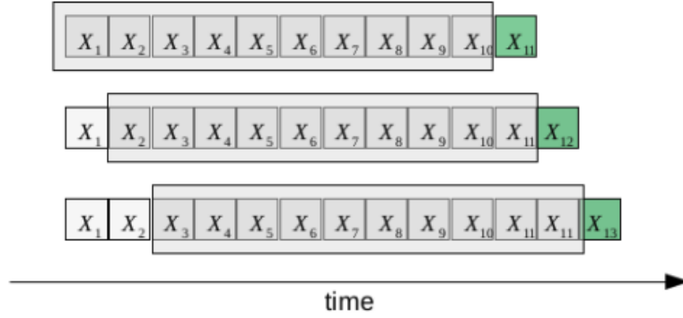
Figura 11: Representación del efecto de una ventana deslizante con LB=10 [2].
