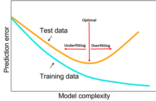
Figura 4.5: Gráfico explicativo de la relación entre el error de entrenamiento ( E_{in} ) y el error de test E_{out} [35].
