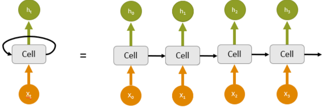
Figura 5.1: Representación de una neurona recurrente y su desglose en el tiempo [50]
