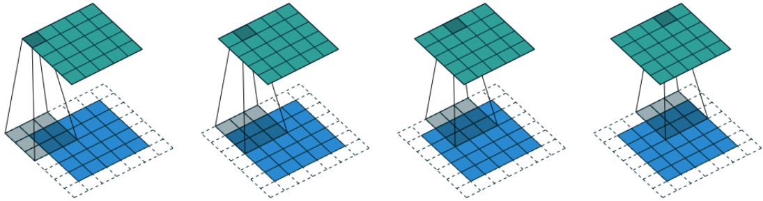
Figura 6.1: Ejemplo de capa convolucional 5 \times 5 con entradas 5 \times 5 con un perímetro de zero padding [55].
