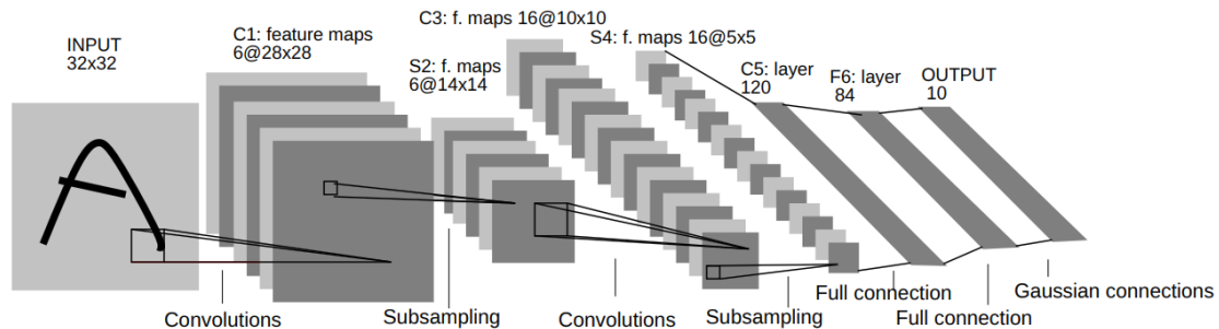
Figura 6.3: Ejemplo de una arquitectura CNN con capas convolucionales y de agregación intercaladas [56]
