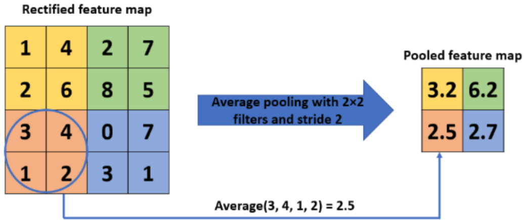
Figura 6.2: Ejemplo de capa pooling basada en la media aritmética de las celdas del campo visual con kernel 2x2 y stride 2 [57].
