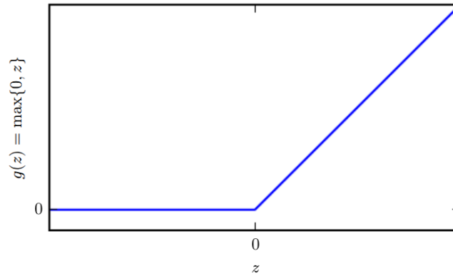
Figura 4.2: Función linear rectificada ReLU(z) [22].
