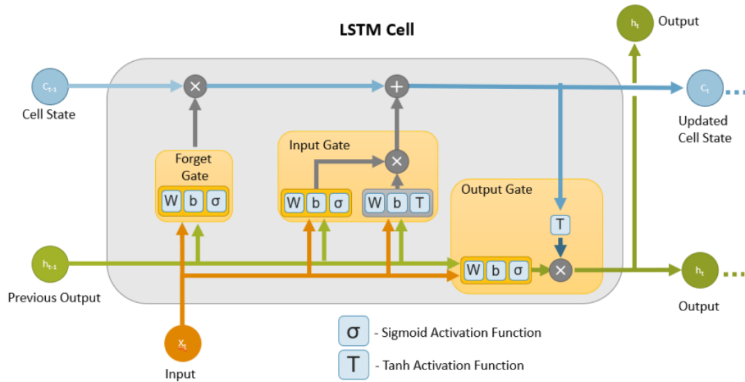
Figura 5.2: Representación de una neurona LSTM con todas sus elementos, puertas y operaciones [50].
