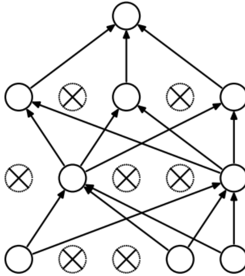
Figura 4.6: Ejemplo de un MLP con dropout durante el entrenamiento [28].
