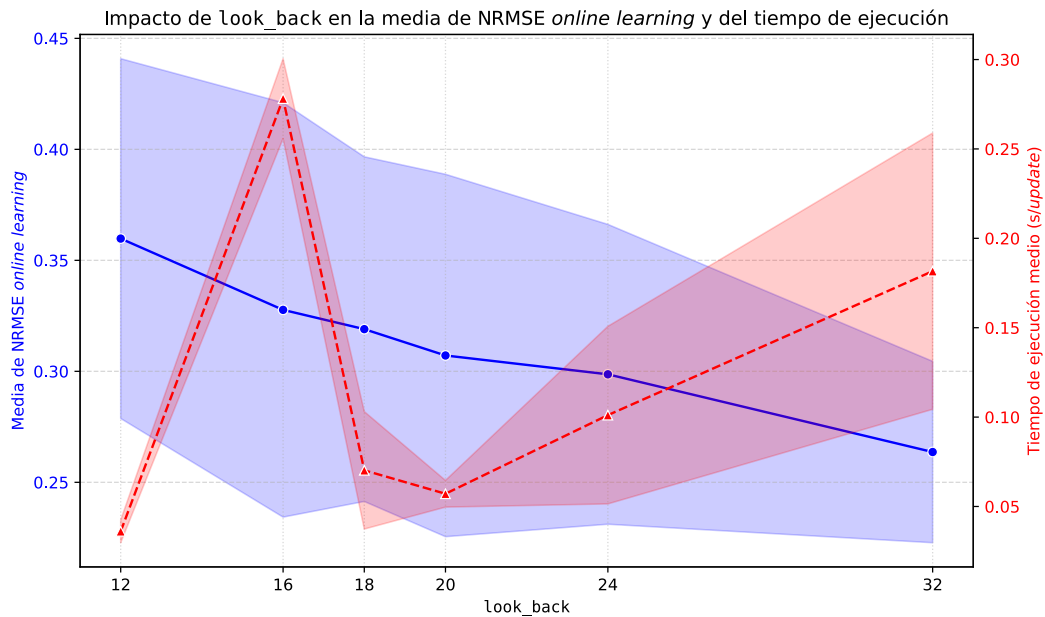
Figura 8.4: Influencia del hiperparámetro look_back en la media del NRMSE y en el tiempo de ejecución medio en modelos con online learning . Elaboración propia.
