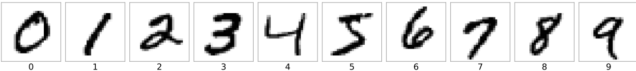
MNIST
