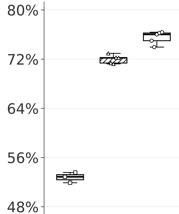
KMNIST
