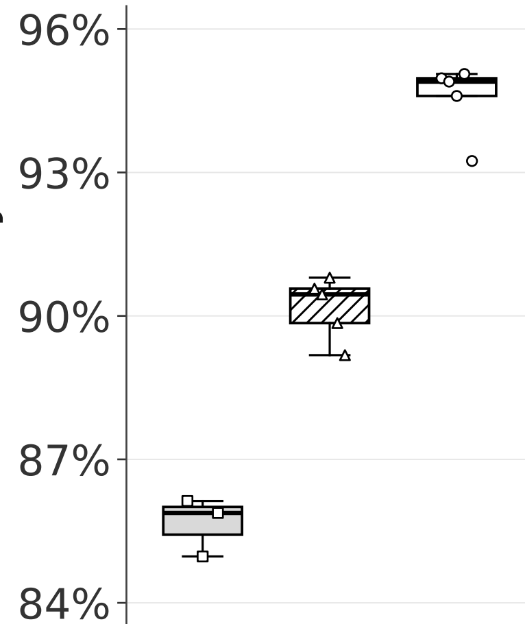
MNIST
