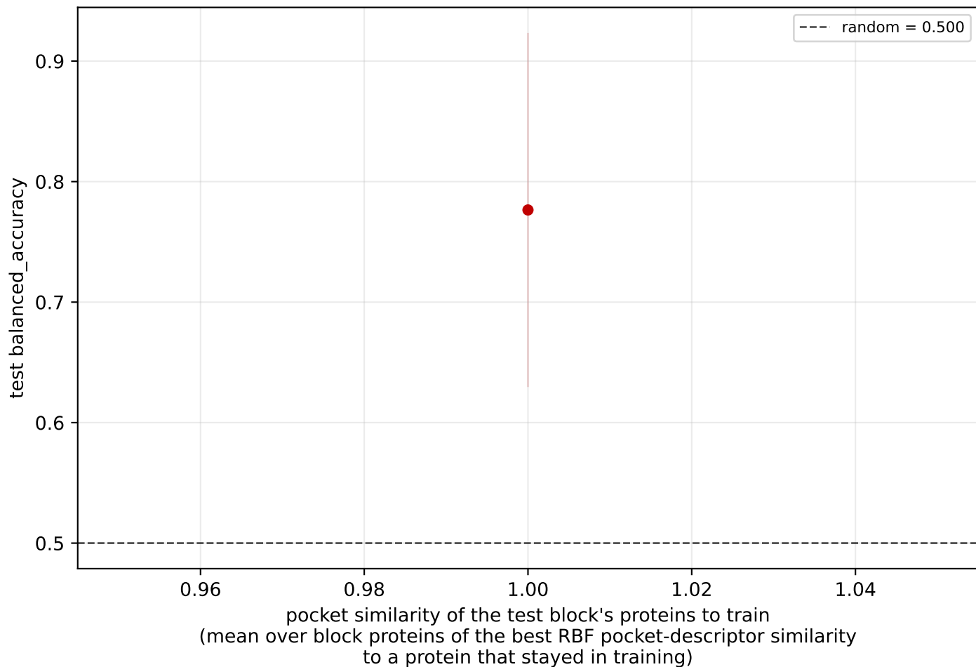
deepclip_f1_normal_mean_cral_trio_iso85_ep120 [lipid_isolation]
