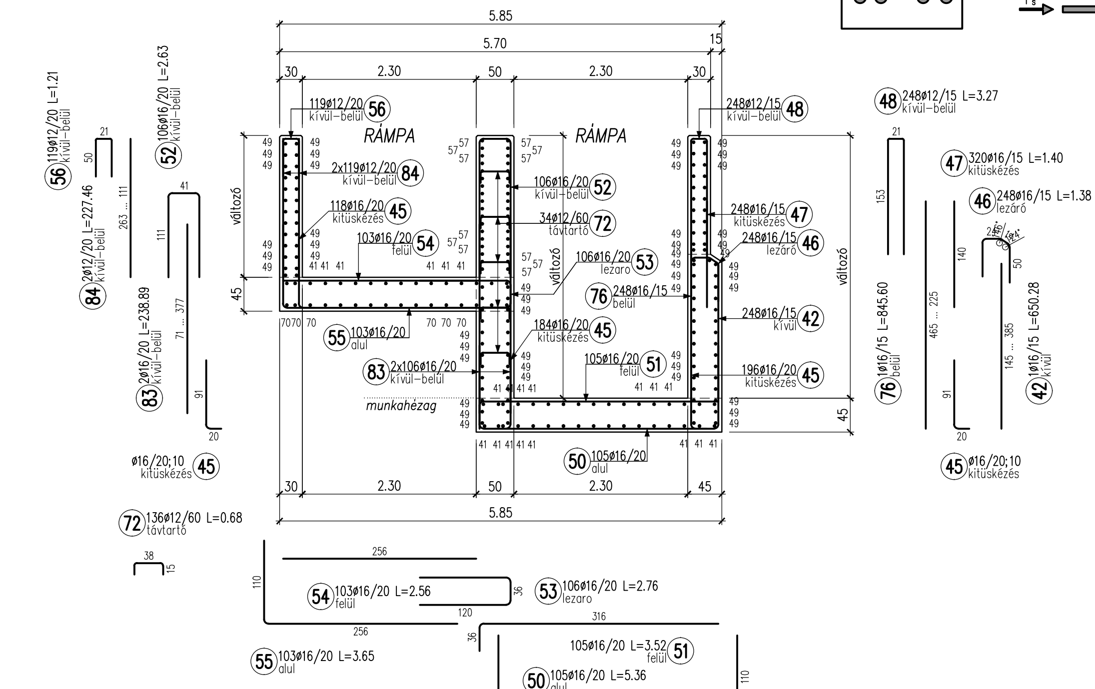
"R-R" KERESZTMETSZET 1:50
