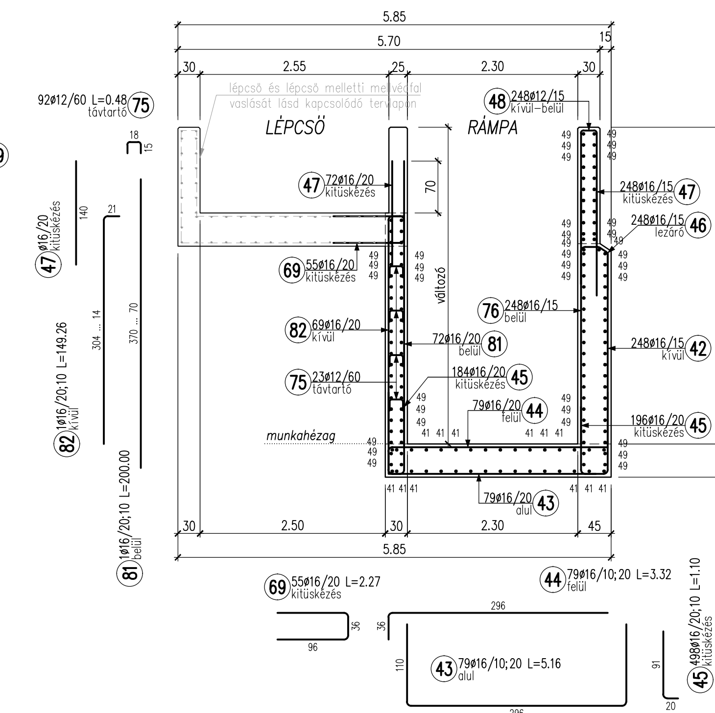
LR-LR JELÜ KERESZTMETSZET 1:50
