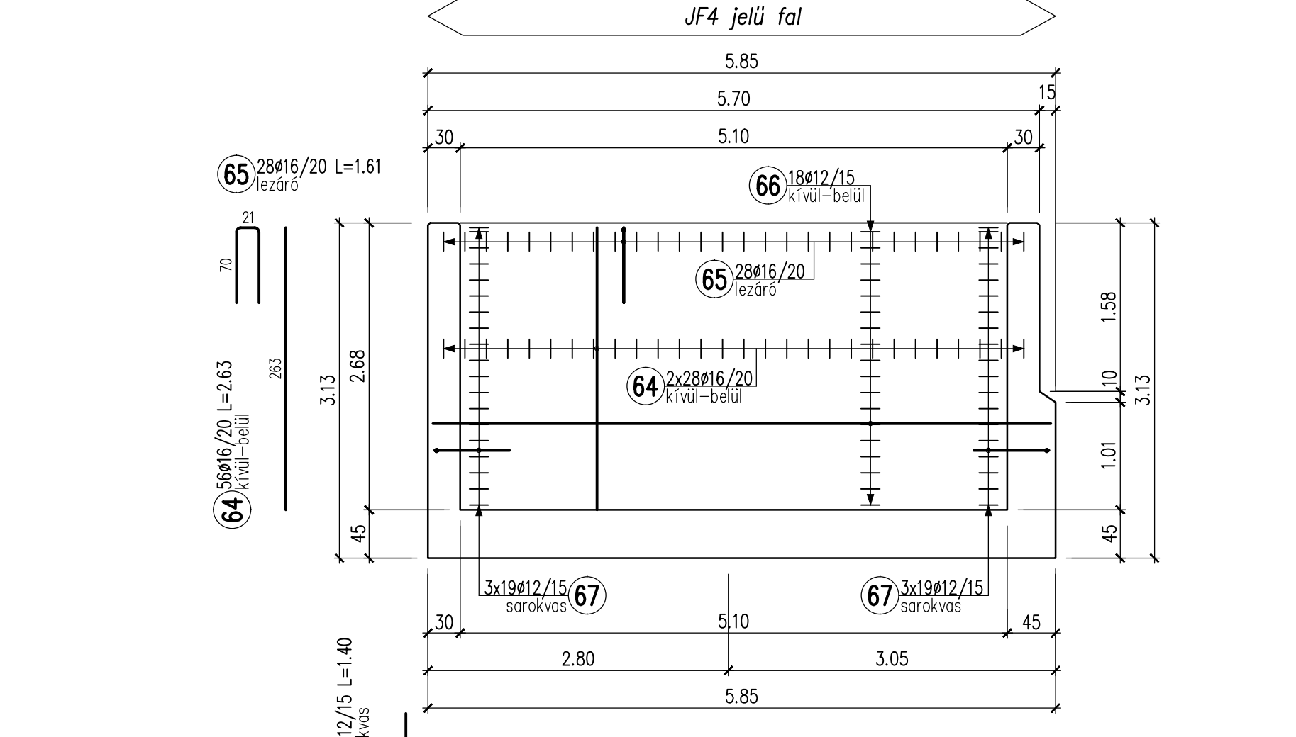
JF4 JELÜ FAL BELSÖ NÉZETE 1:3
