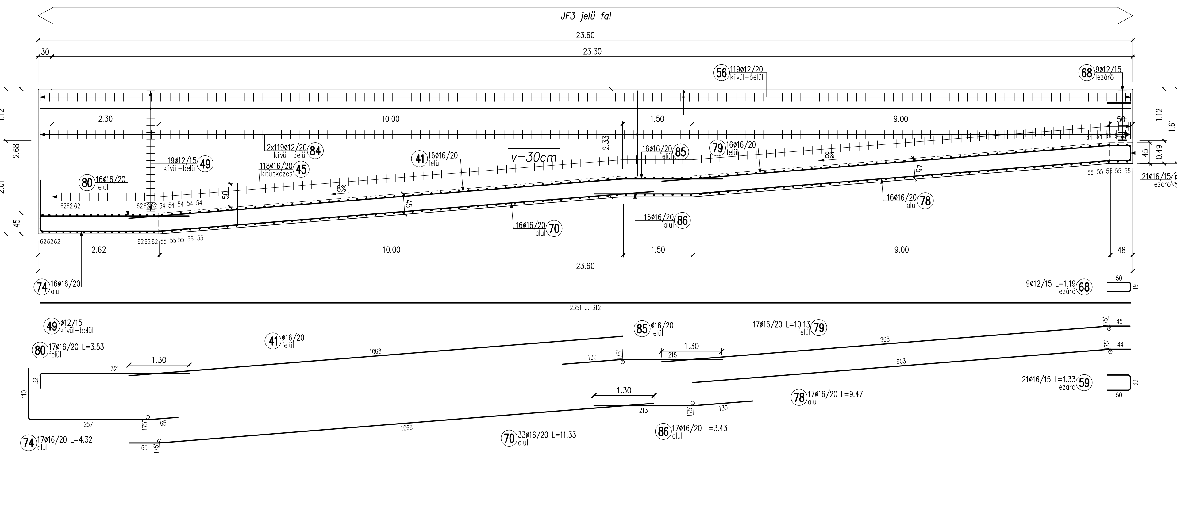
JF3 JELÜ FAL KÜLSÖ NÉZETE 1:50
