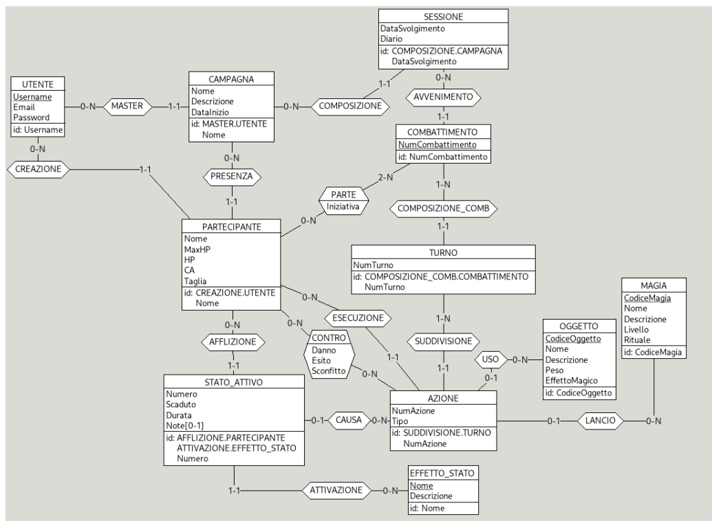
Figura 2.10: Combattimento, Effetti di stato e Statistiche
