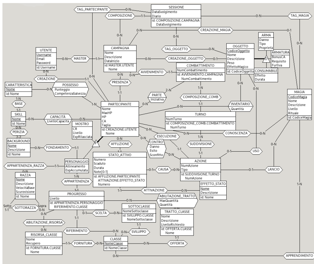
Figura 2.11: Schema concettuale finale
