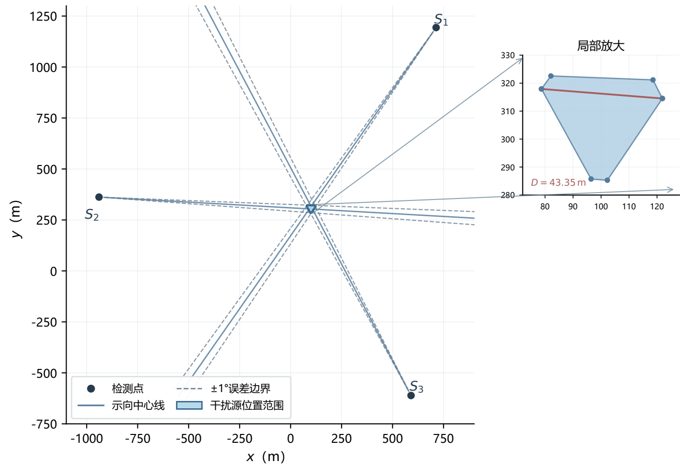
检测点示向交会示意图
