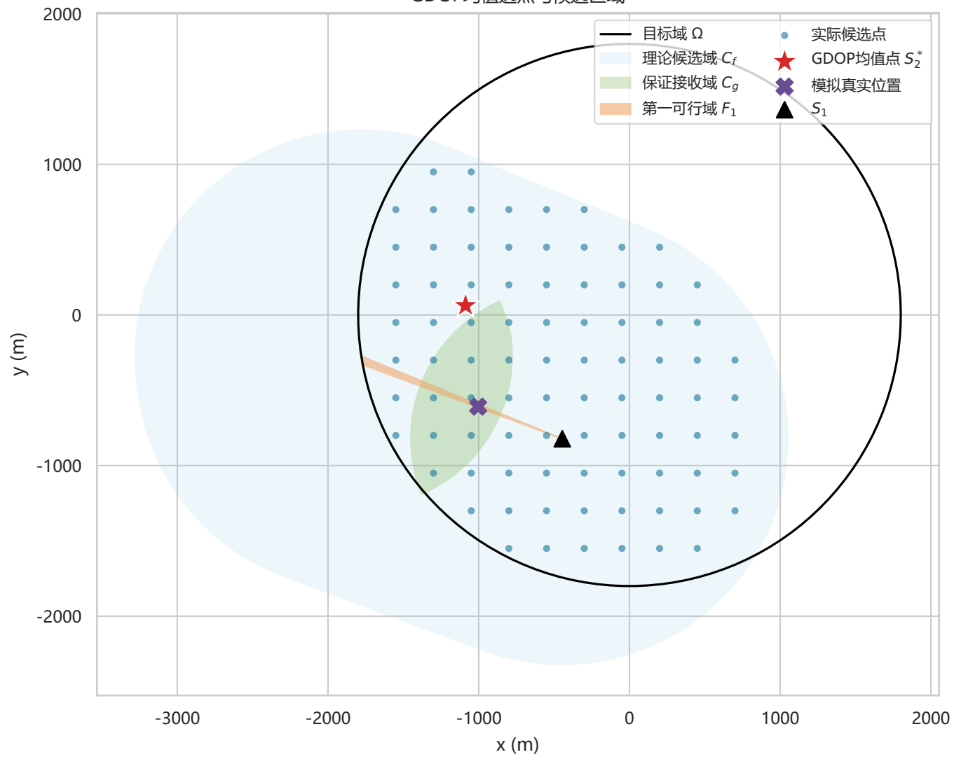
GDOP均值选点与候选区域
