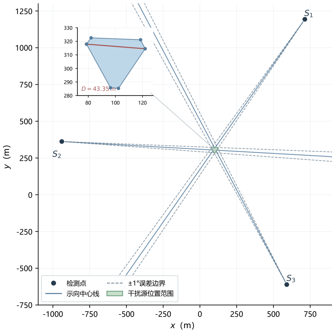
检测点示向交会示意图
