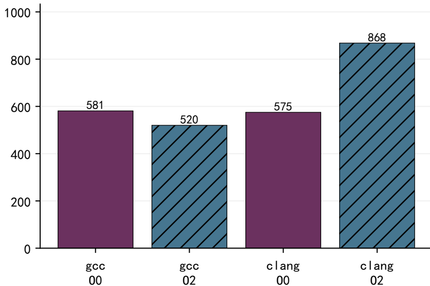
可执行文件 .text 段 (字节)
