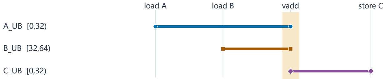
(b) 内容活跃区间：首次写入 → 最后读取
