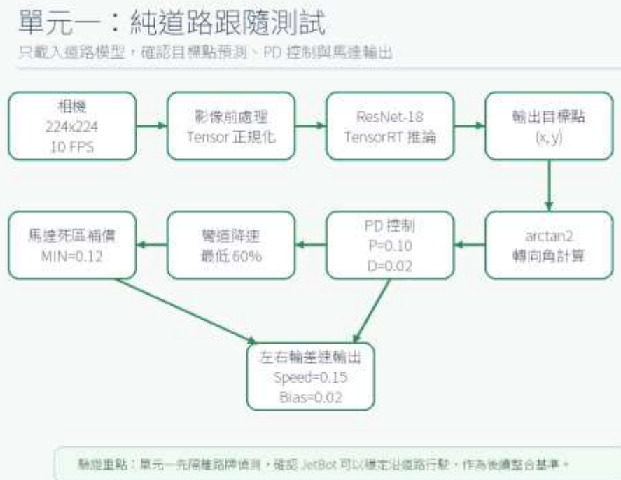
圖 10：單元一道路跟隨控制流程
