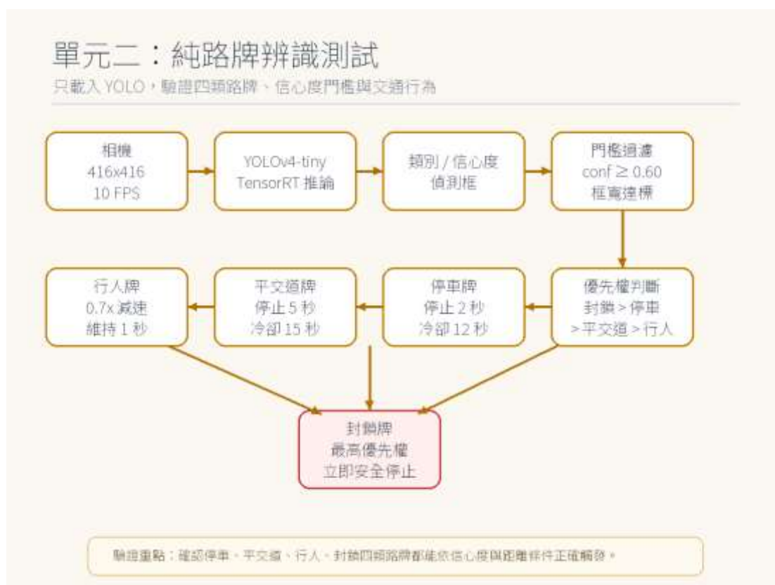
圖 12：單元二路牌辨識控制流程
