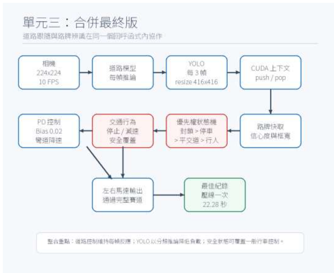
圖 14：單元三最終整合控制流程
