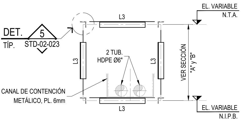
SECCIÓN D-D (VER NOTA 4) ESC.:1/25
