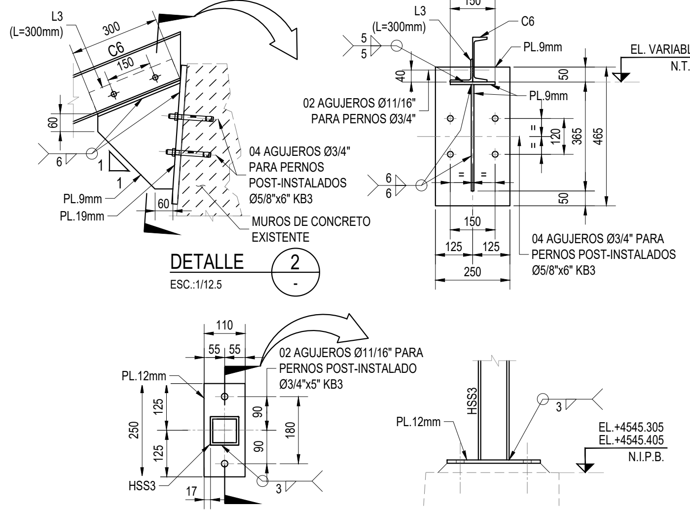
DETALLE DE PLACA BASE PB-1 - PLANTA
