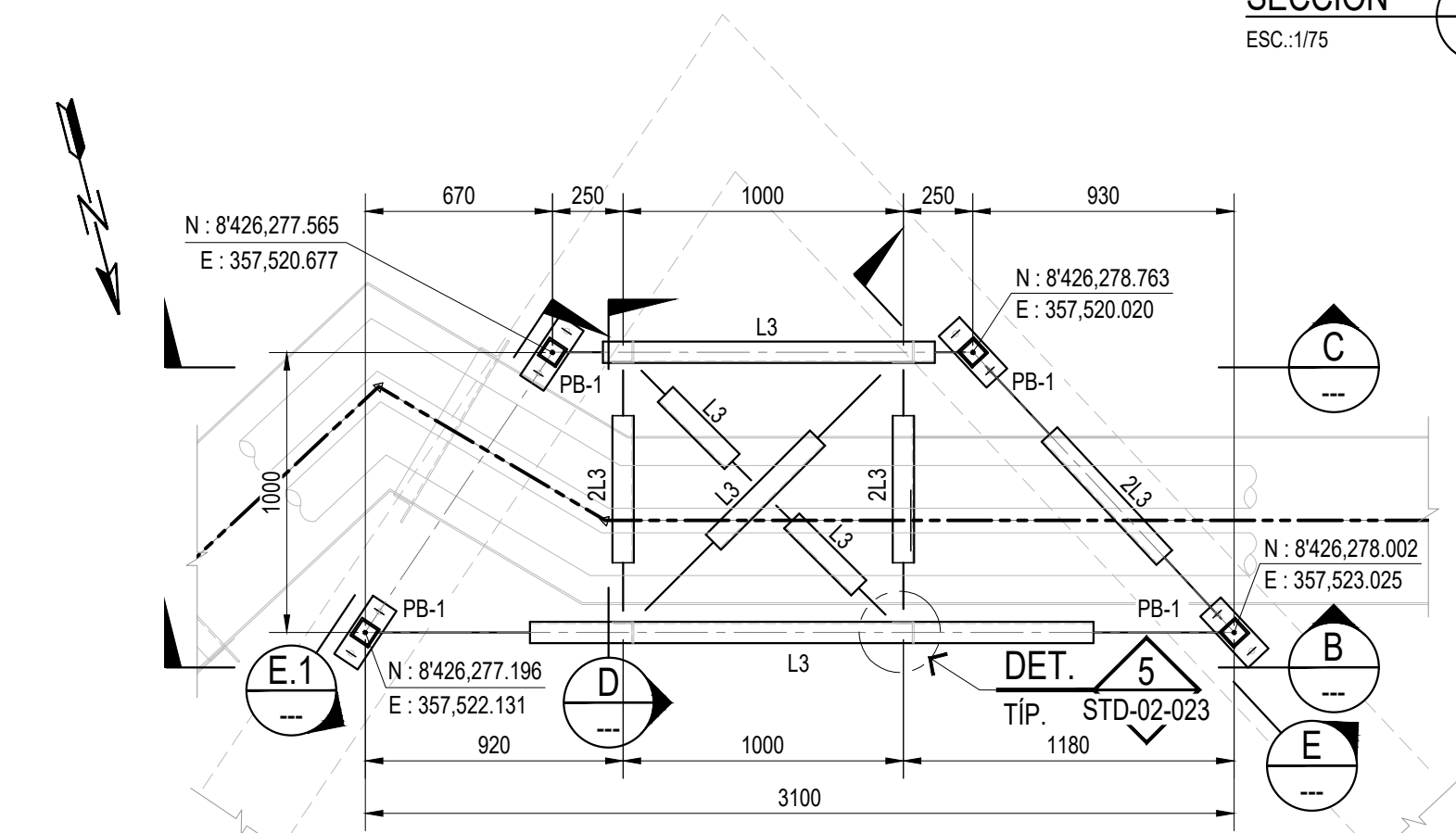
DETALLE 1 (VER NOTA 4) ESC.:1/25
