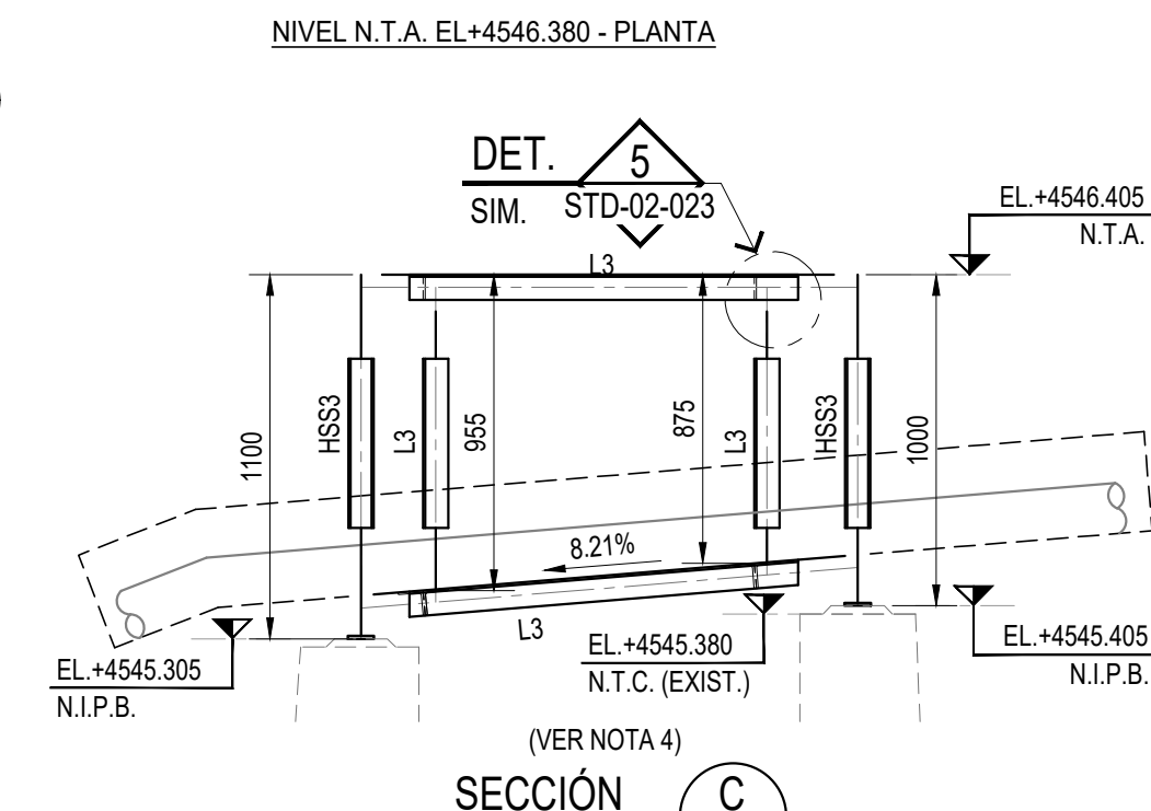
SECCIÓN C-C (VER NOTA 4) ESC.:1/25
