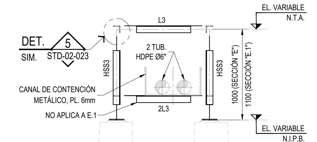
SECCIÓN E-E (VER NOTA 4) ESC.:1/25
