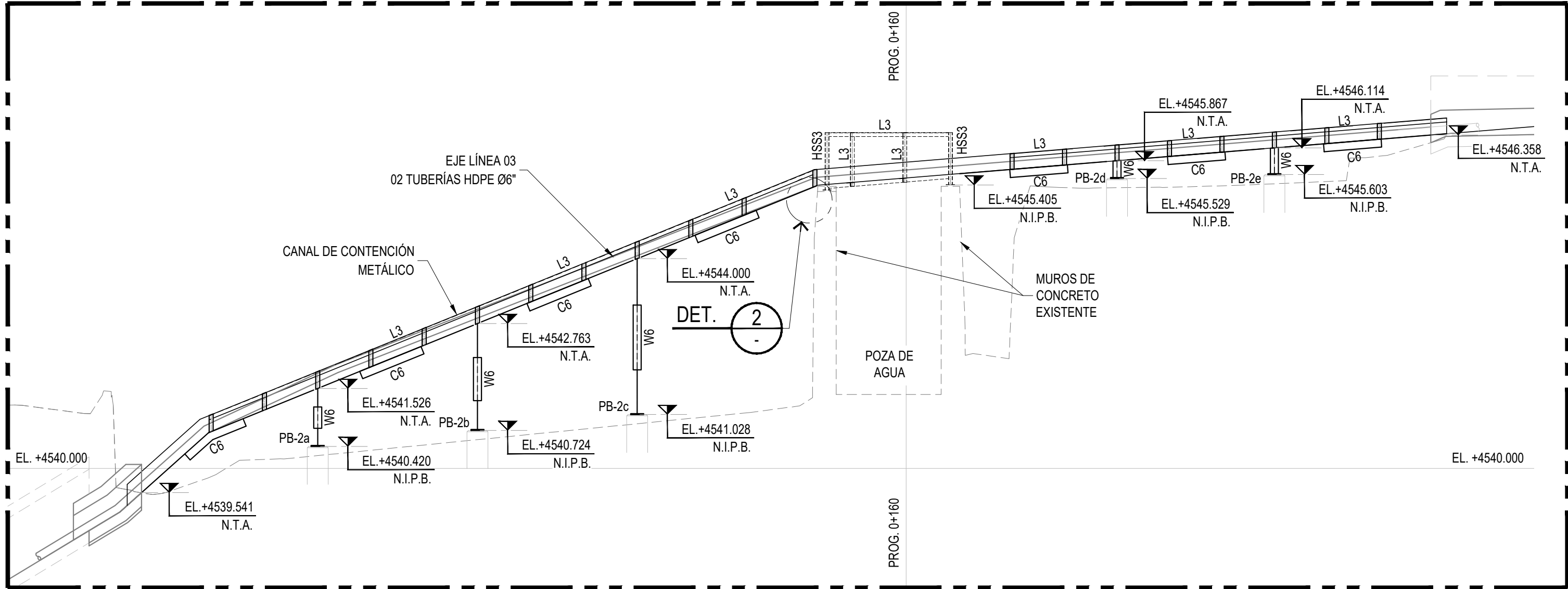
SECCIÓN A-A (VER NOTA 4) ESC.:1/75
