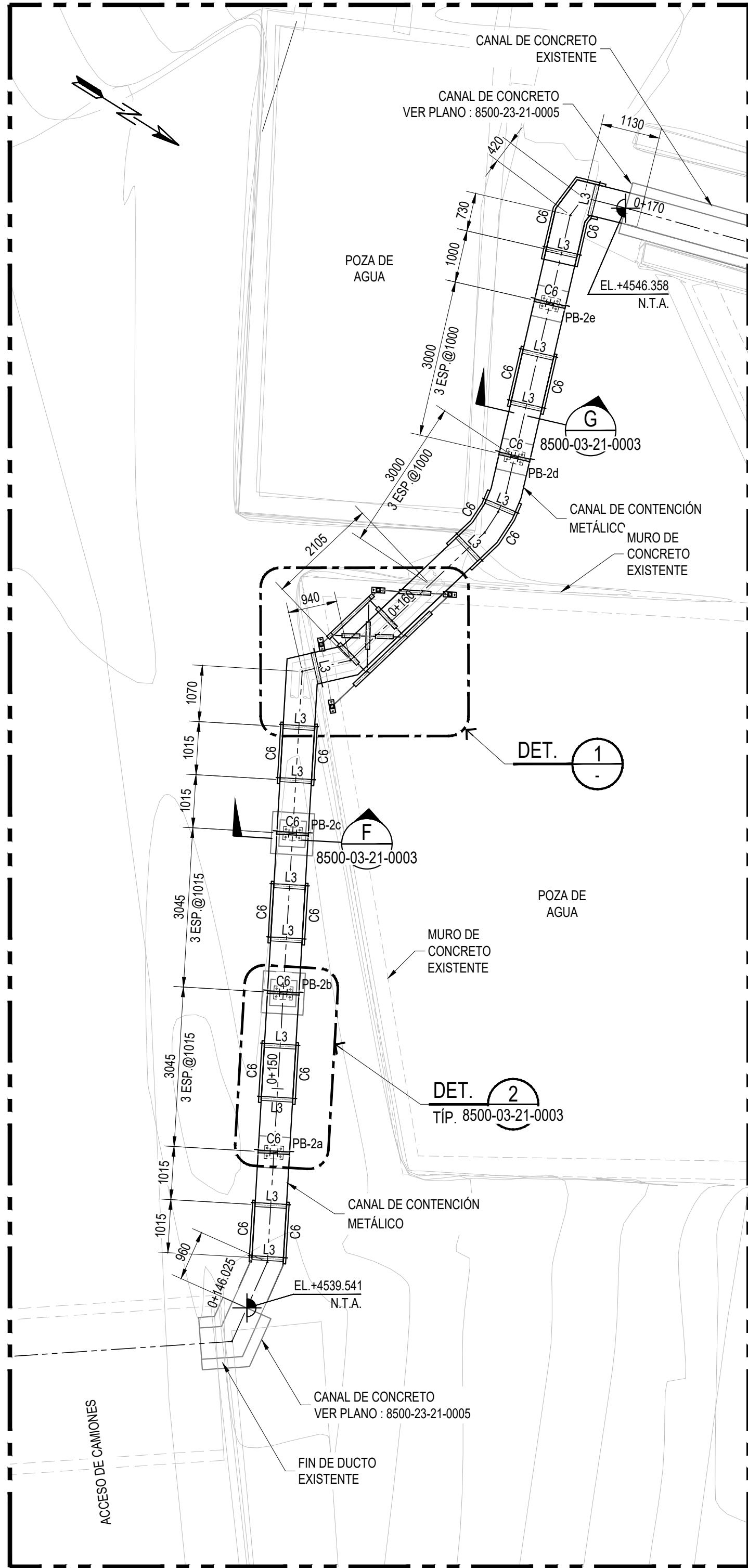
SISTEMA DE CONTENCIÓN LÍNEA 03 - PLANTA (S/C=180 Kg/m 2 ) PROGRESIVA 0+146.025 A 0+170 ESC.:1/75
