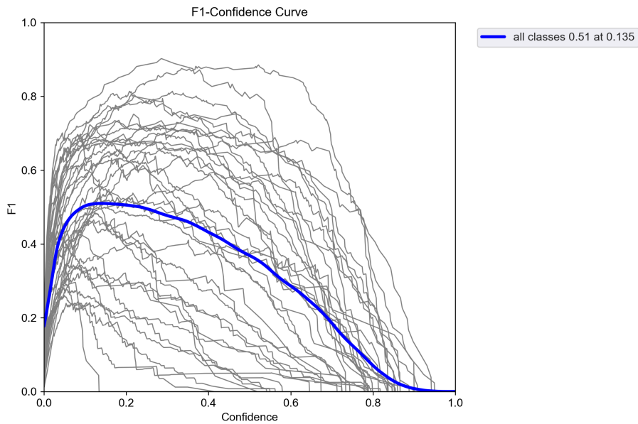
图 5 F1 与置信度阈值关系
