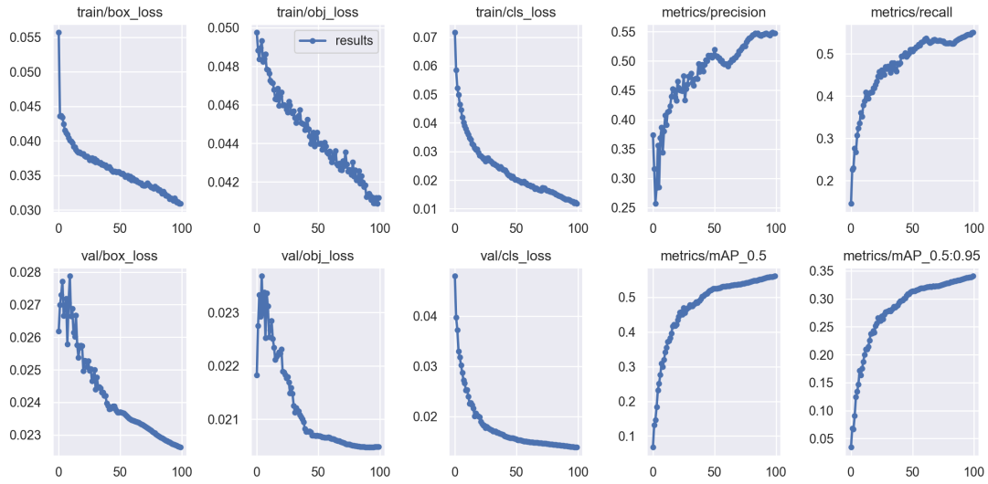
图 4 训练与验证指标变化曲线
