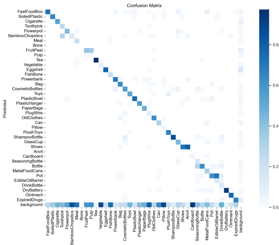
图 7 模型归一化混淆矩阵
