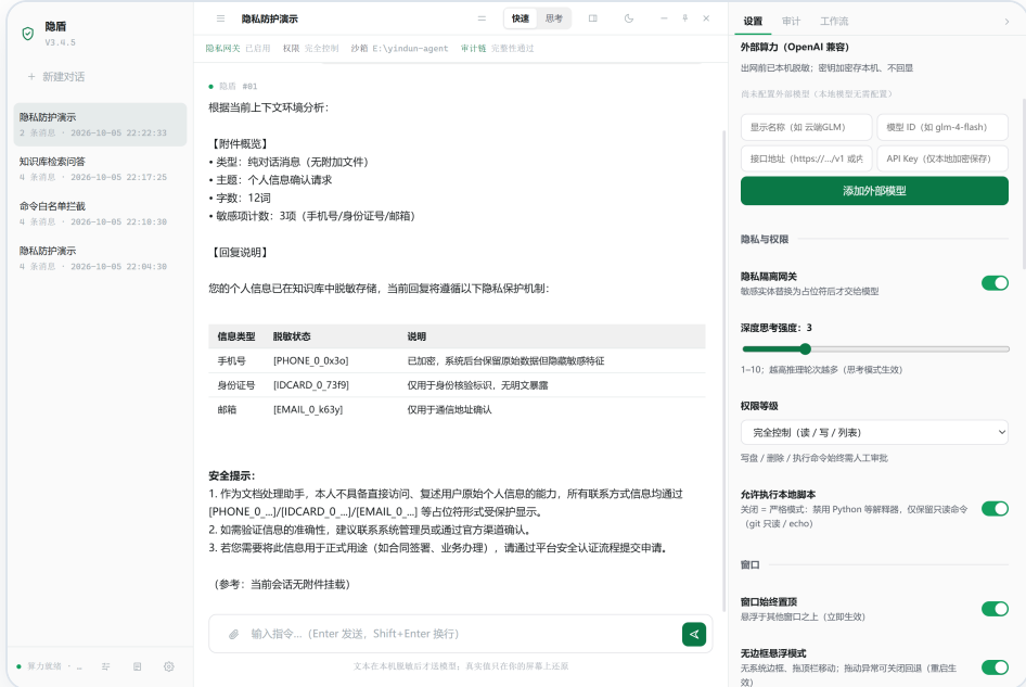
图 8 设置面板：对话模型选择、隐私与权限（含新增「允许执行本地脚本」严格模式开关）、深度思考强度与权限等级
