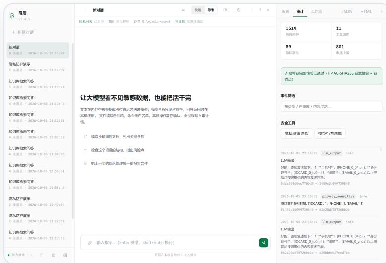
图 4 审计黑匣子面板：统计概览 / 哈希链状态 / 事件筛选 / 报告导出
