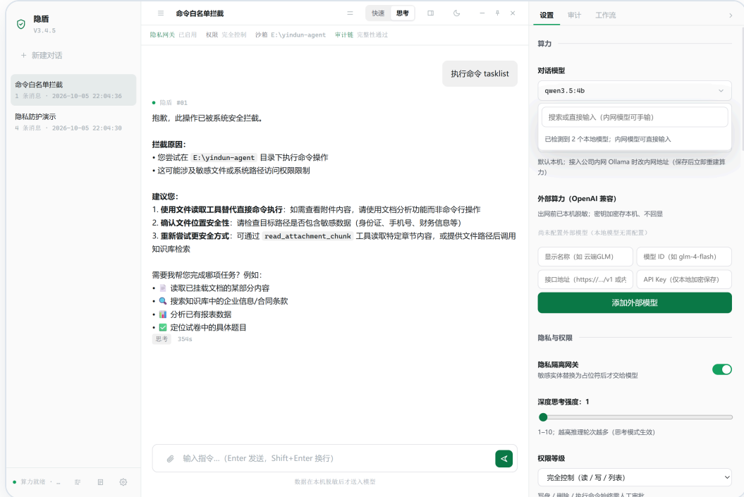
图 5 命令白名单实测：非白名单命令（tasklist）被内核拦截，模型基于真实拦截结果如实反馈（工具决策由受控脚本注入，拦截与回答为真实链路）
