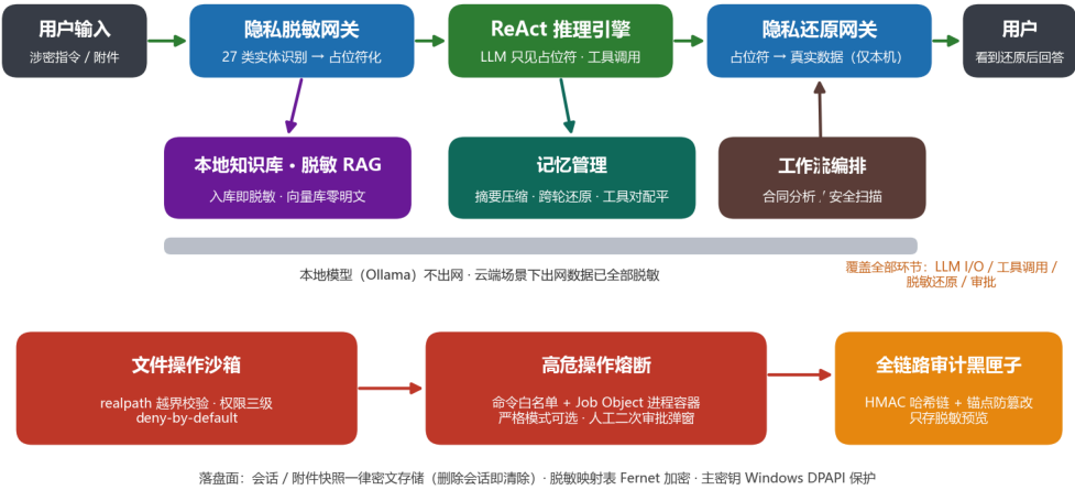
隐盾安全智能体 · 核心数据流与安全防线
