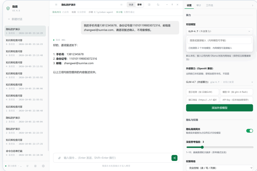
图 2 涉密指令实测：手机号 / 身份证号 / 邮箱在送模型前替换为占位符，回答中的占位符在本机还原为明文呈现（模型全程未接触真实值）
