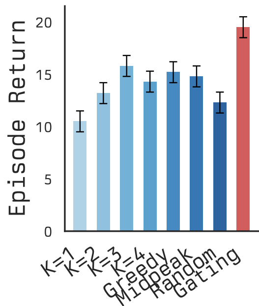
Sokoban
