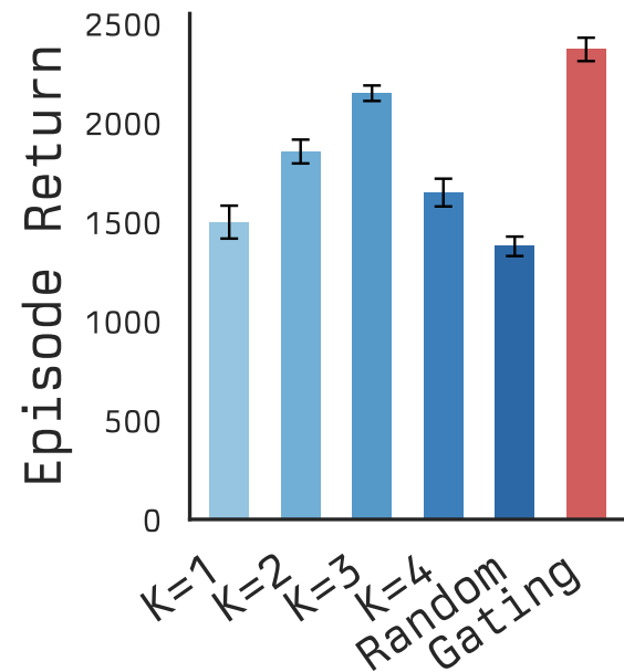
Pac-Man
