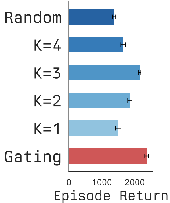
Pac-Man
