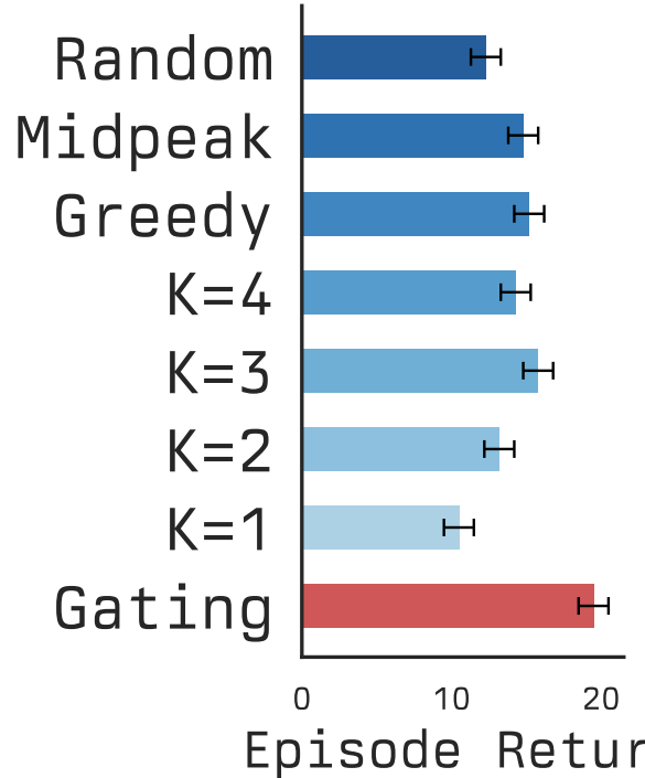
Sokoban
