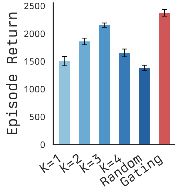
Pac-Man
