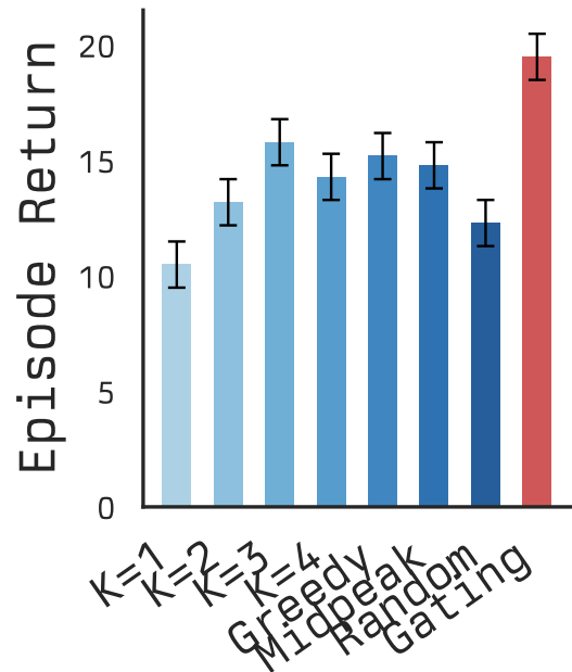
Sokoban
