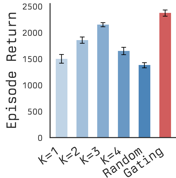
Pac-Man
