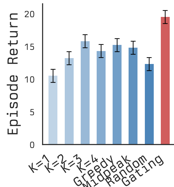
Sokoban
