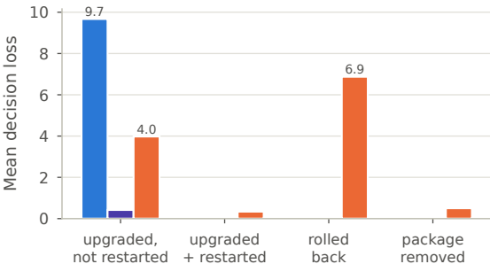
D1 drift (D2 episodes)
