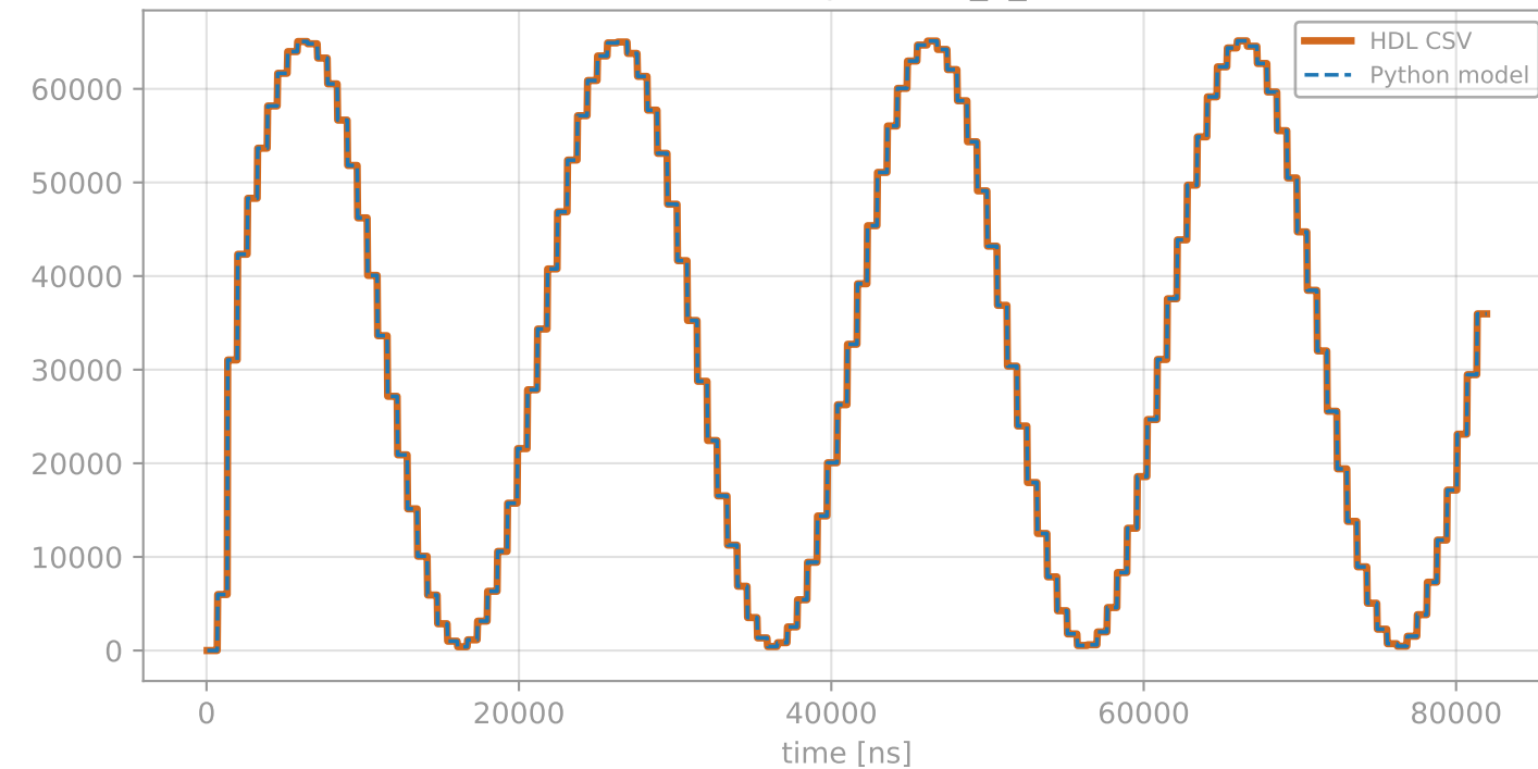
Decimator output (dec_o_data)
