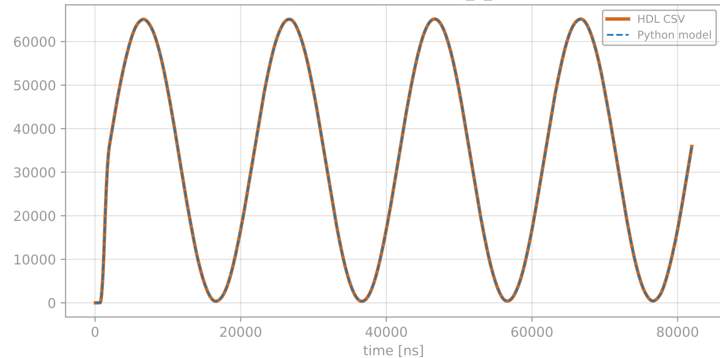
Interpolator output (interp_o_data)
