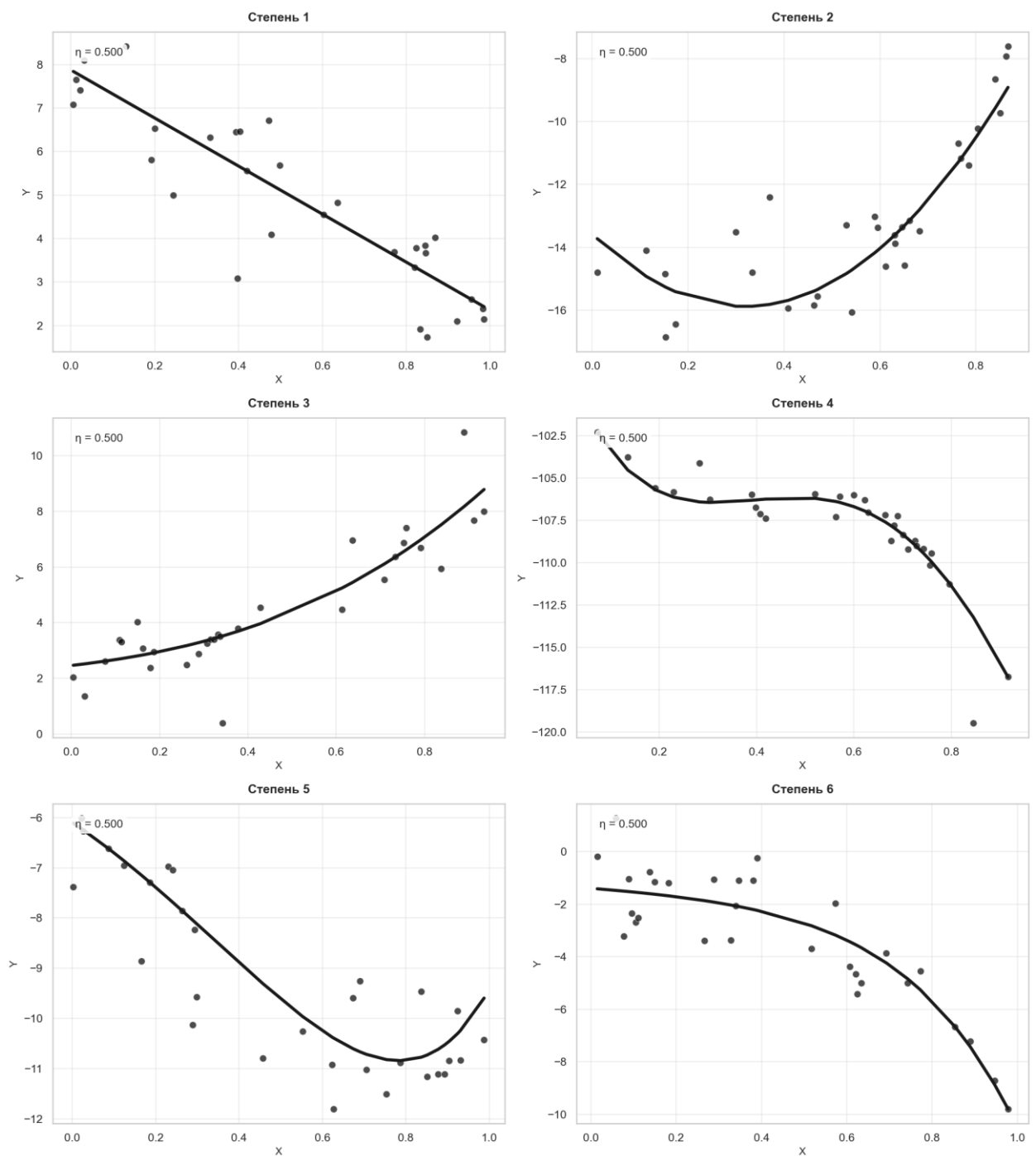
Рисунок 5 — Примеры датасетов при высоком относительном уровне шума
