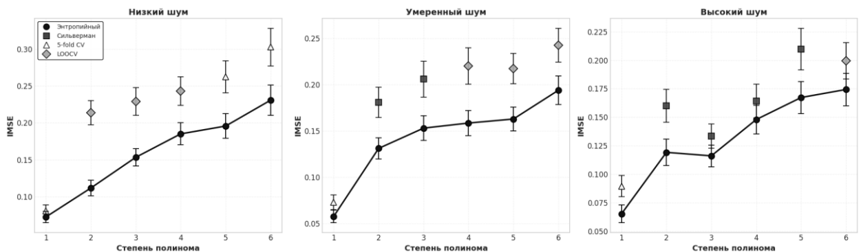
Рисунок 31 — Сравнение методов регрессии: IMSE в зависимости от степени полинома
