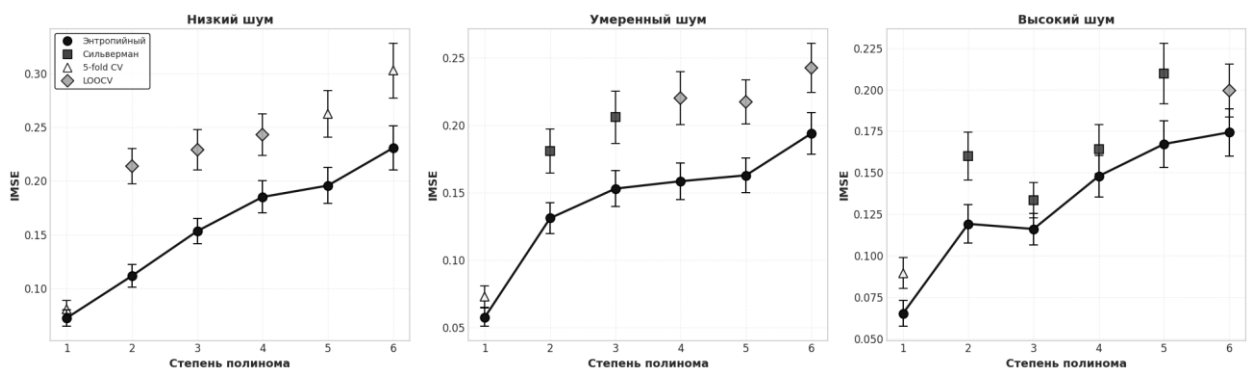
Рисунок 35 — Сравнение методов регрессии: IMSE в зависимости от степени полинома
