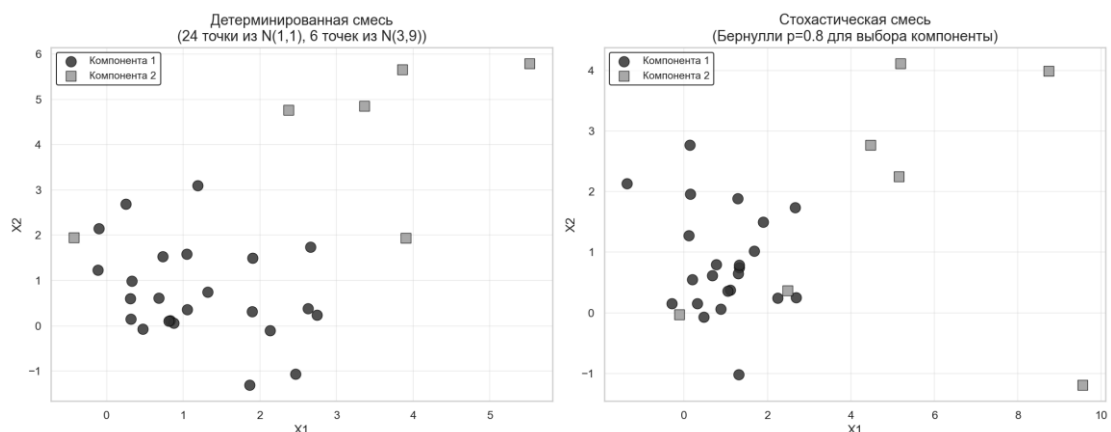
Рисунок 14 — Примеры генераций смеси распределений
