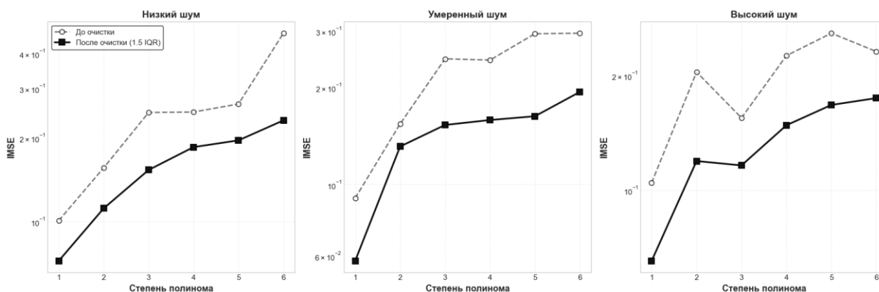
Рисунок 31 — Влияние IQR-очистки на IMSE: энтропийный метод
