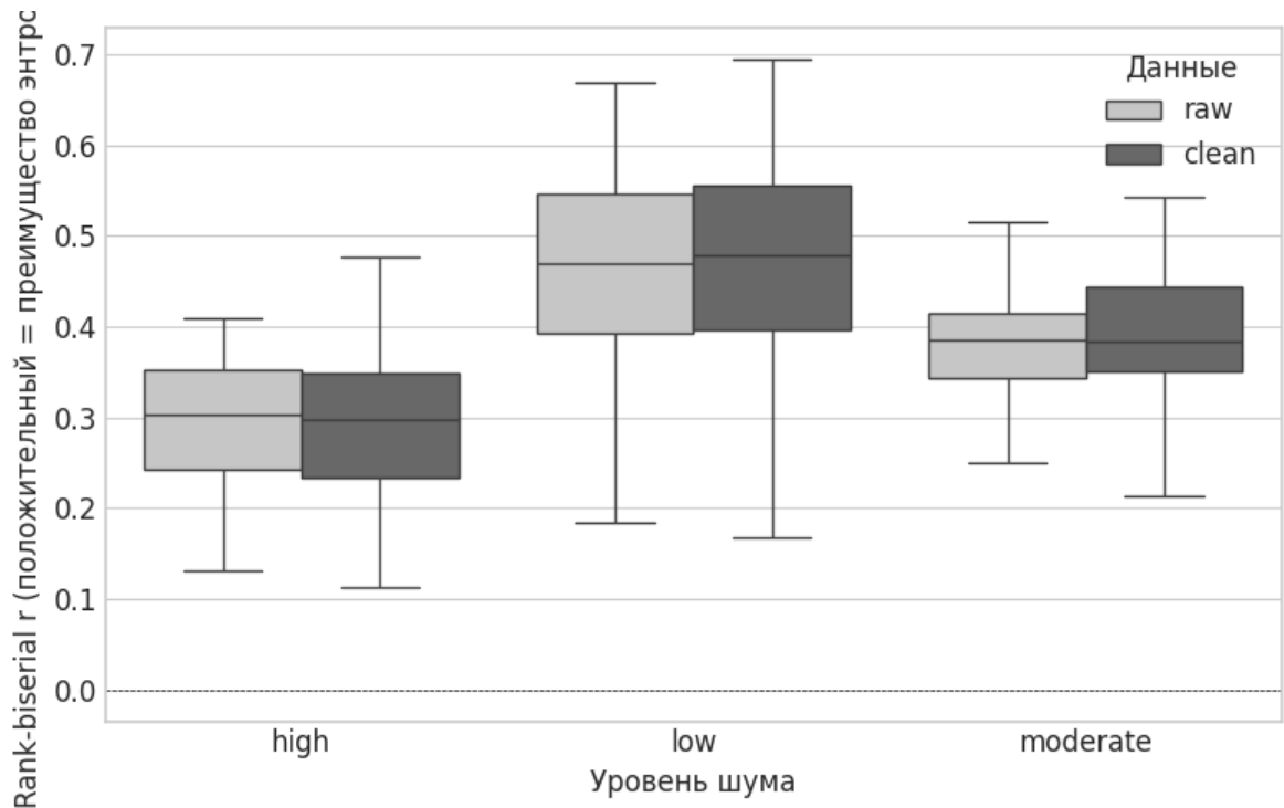
Рисунок 34 — Размер эффекта (rank-biseral) во всех конфигурациях
