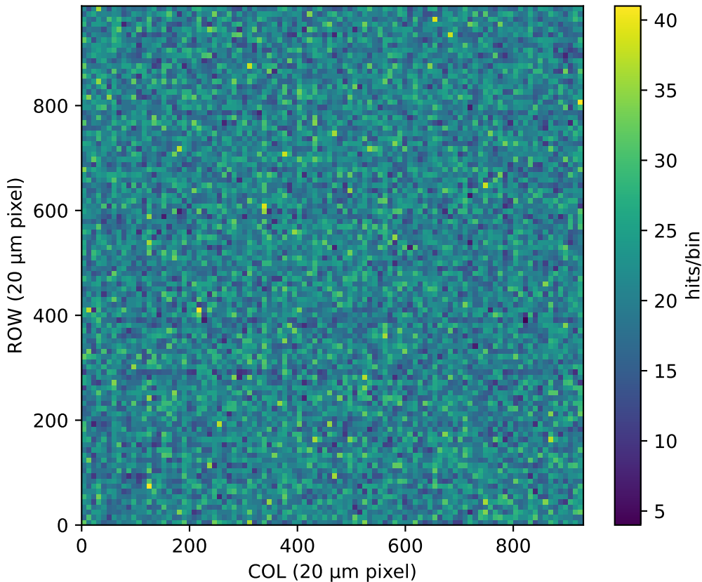
VTXOB layer 4 occupancy (204698 hits)
