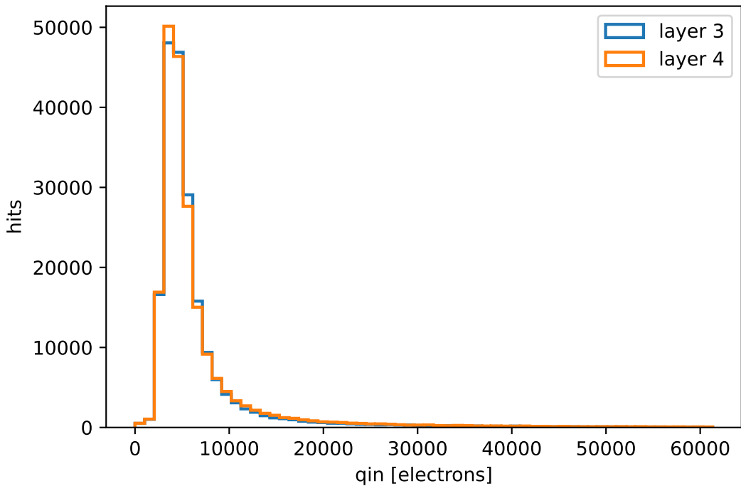
Charge (median 4788 e-, MIP~3600)
