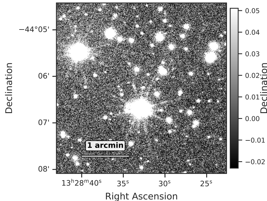
(d) Central Region - Original
