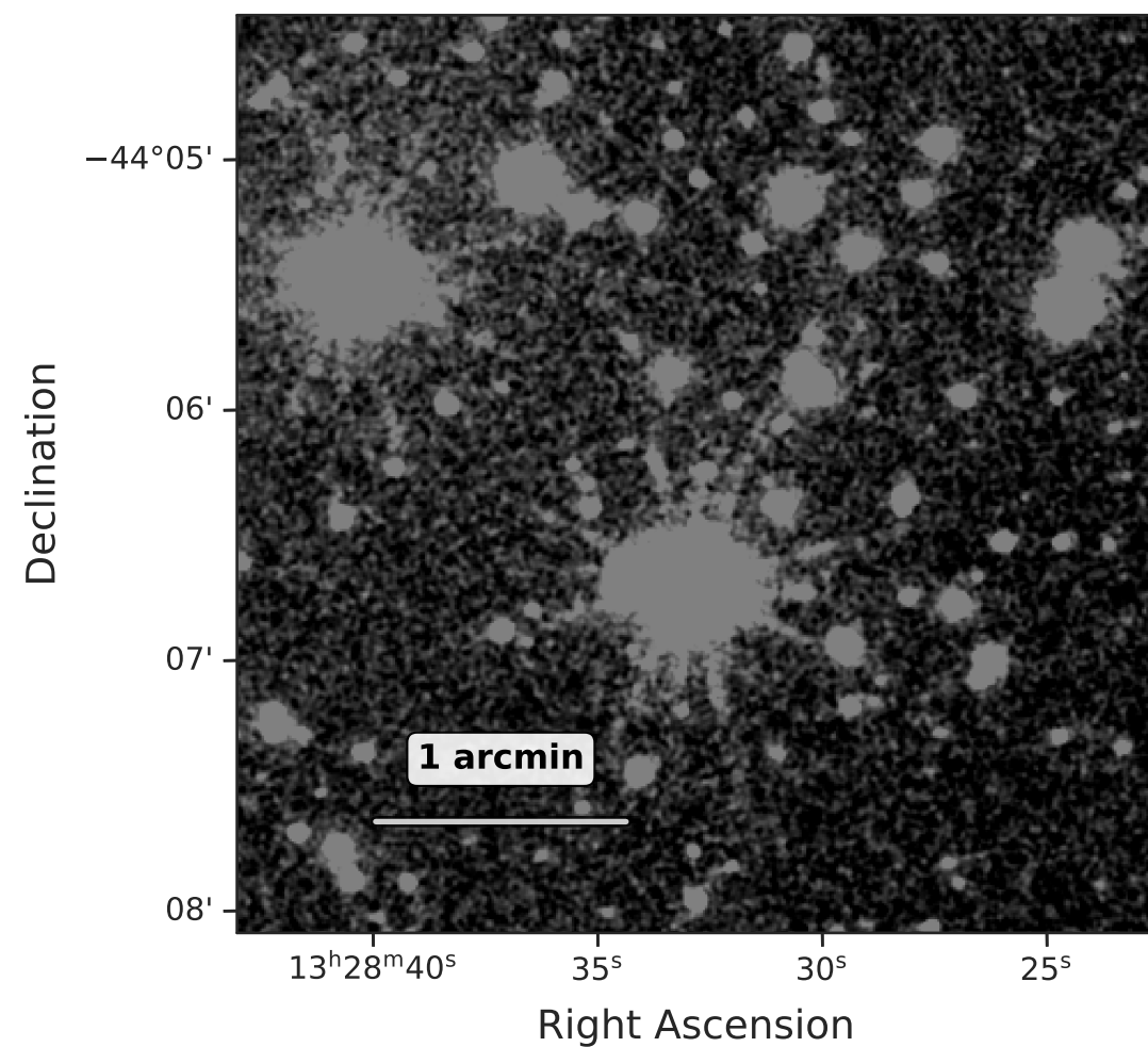
(d) Central Region - Enhanced
