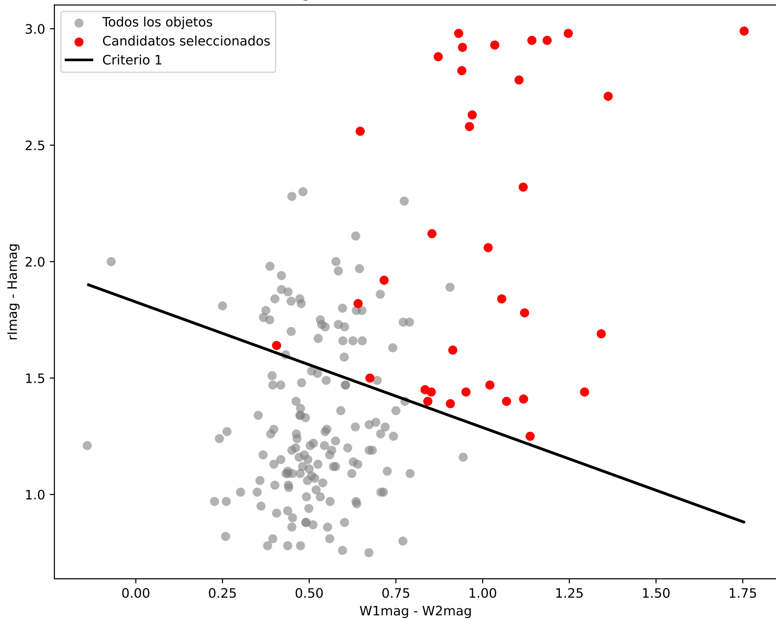
Diagrama de Color-Color (Criterio 1)
