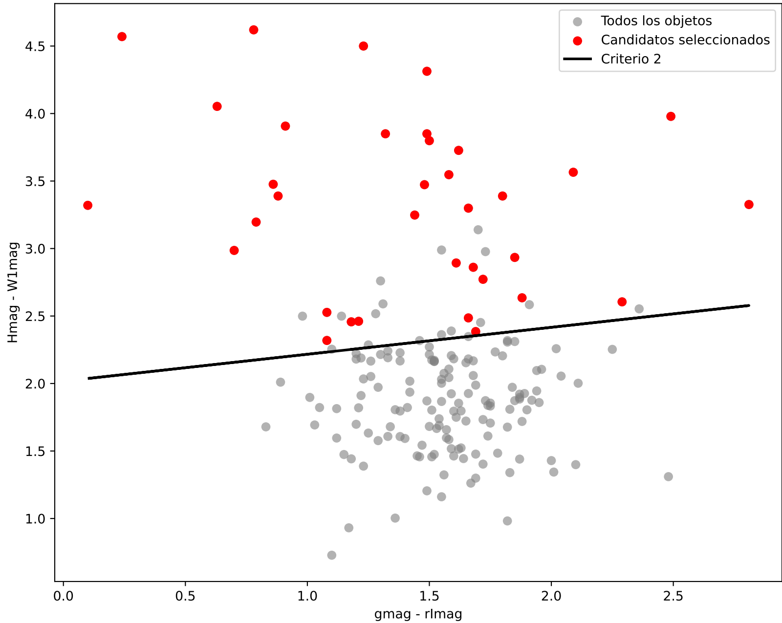
Diagrama de Color-Color (Criterio 2)
