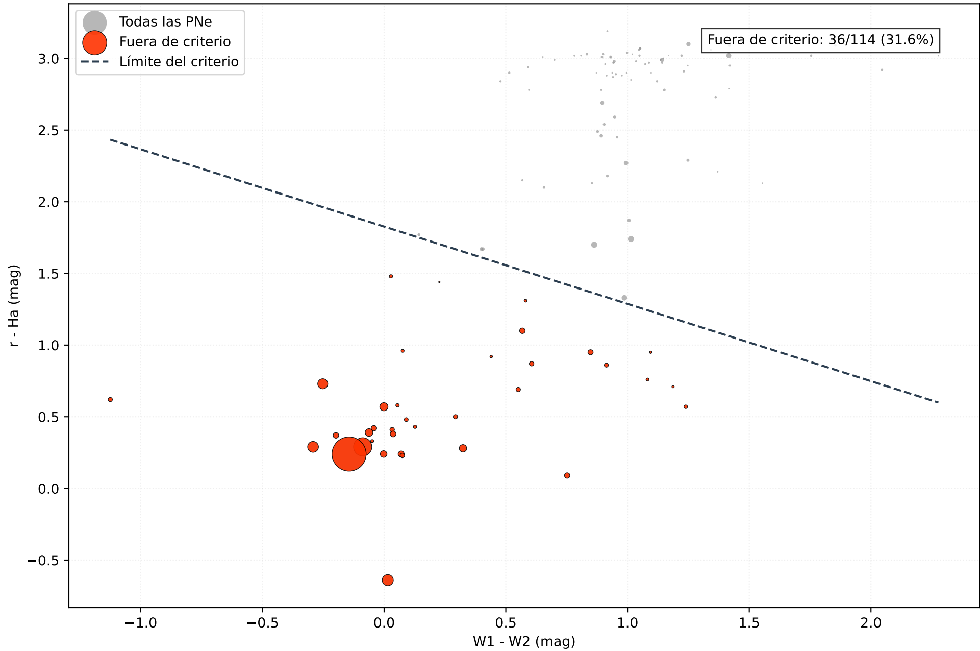
Criterio 1: W1-W2 vs r-H \alpha
