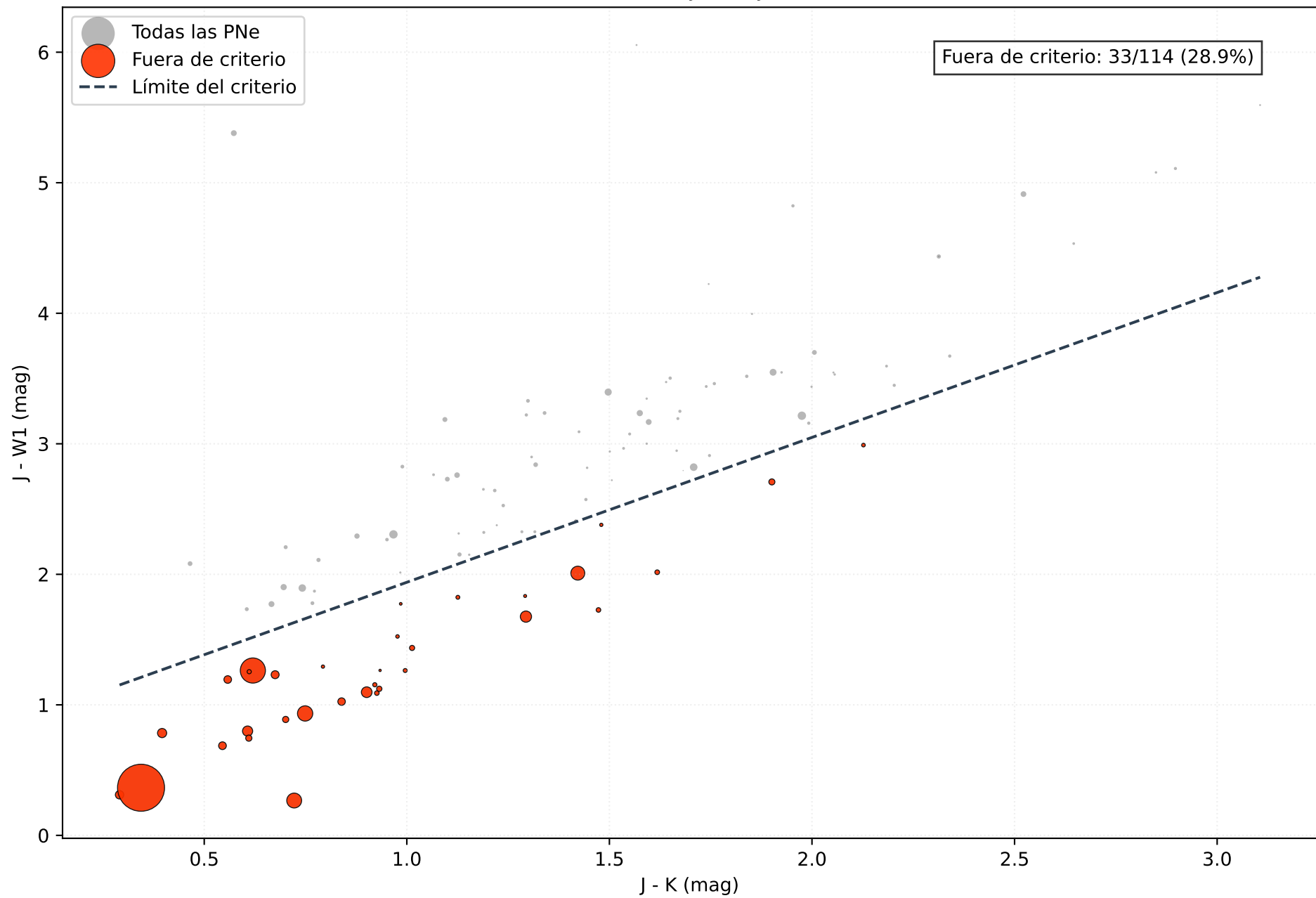
Criterio 7: J-K vs J-W1
