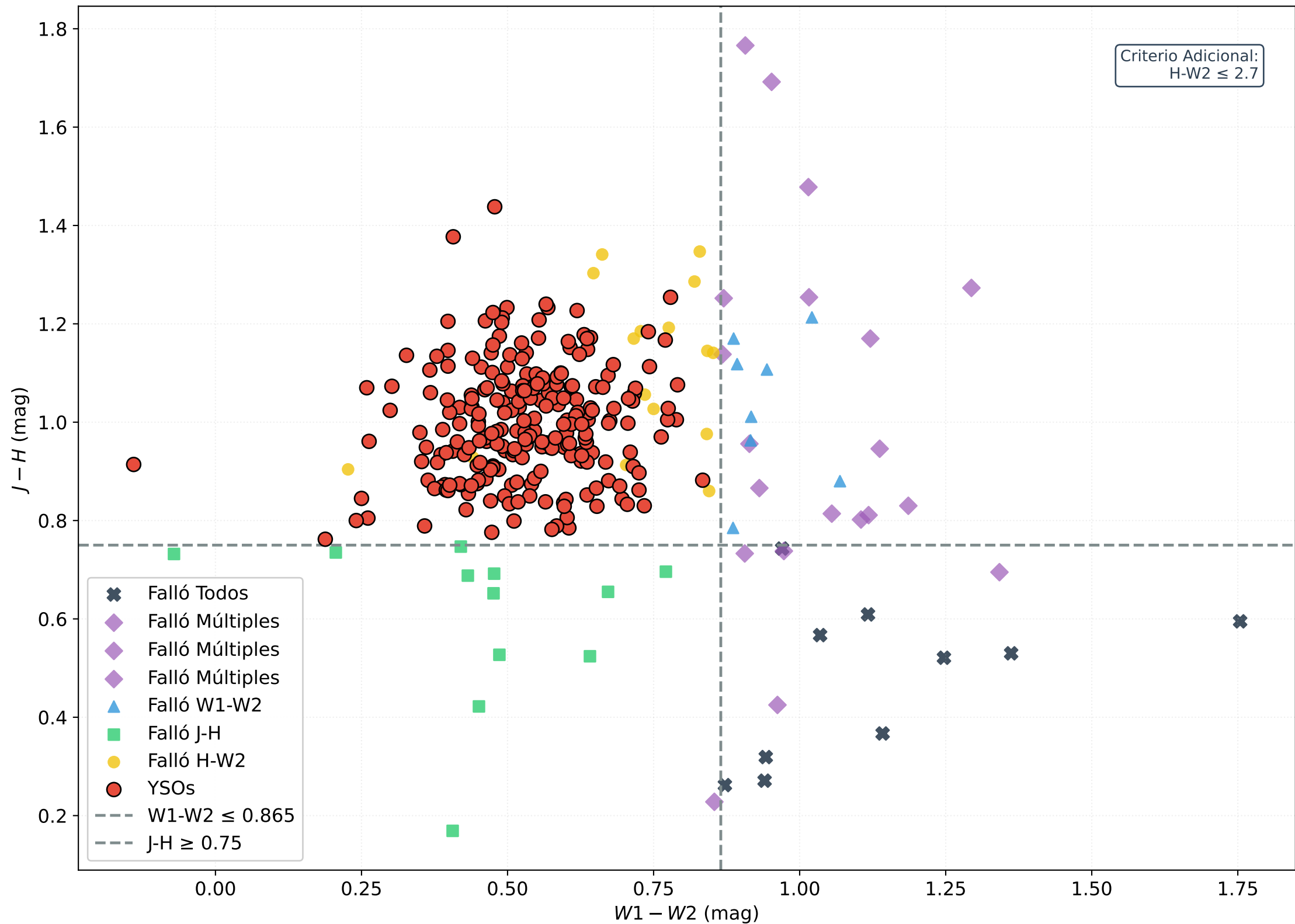
Clasificación YSO/PNe: W1-W2 vs J-H (Criterio H-W2 no visible)
