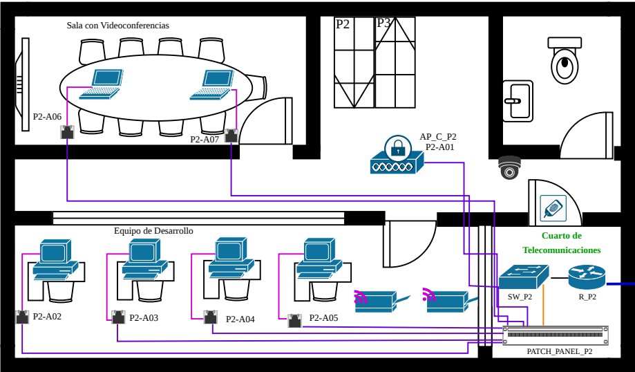
SEGUNDO PISO (P2)
