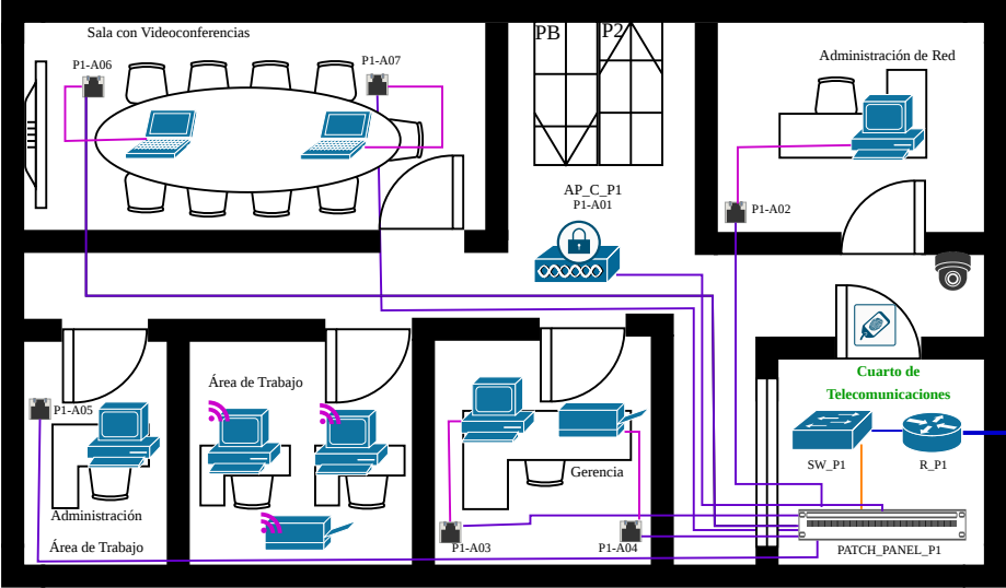
PRIMER PISO (P1)
