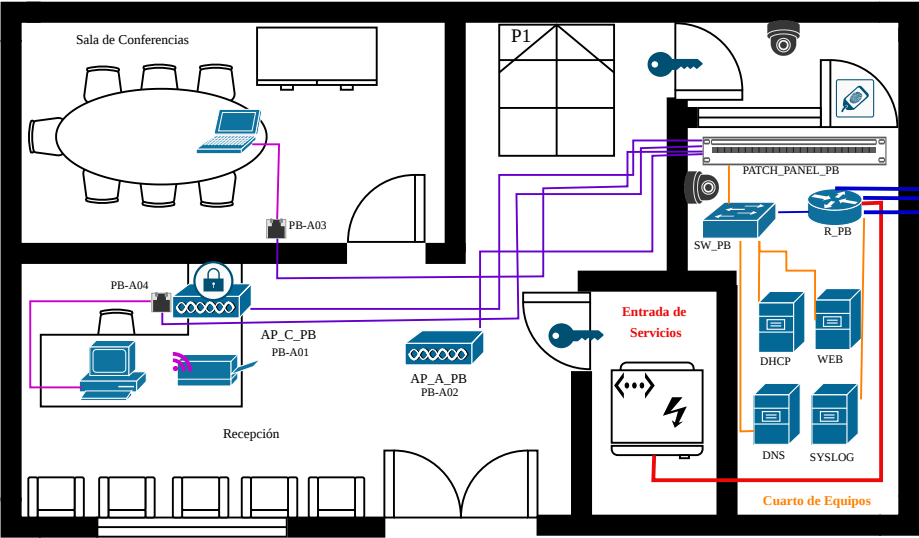
PLANTA BAJA (PB)
