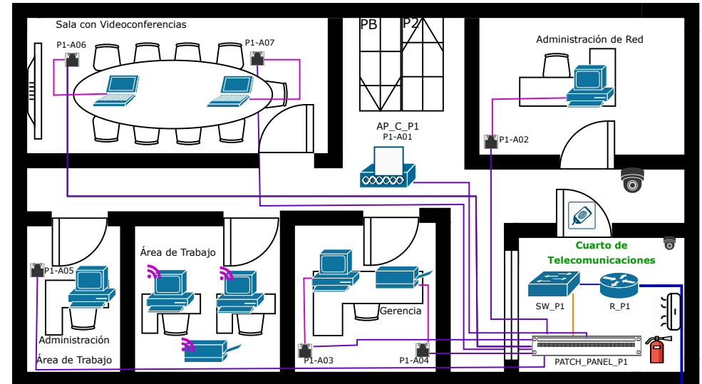
PRIMER PISO (P1)
