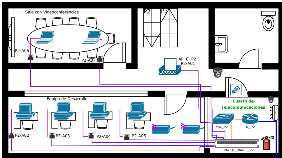
SEGUNDO PISO (P2)
