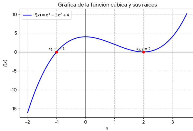
Figura 5: Gráfica de la función cúbica señalando la raíz repetida.
