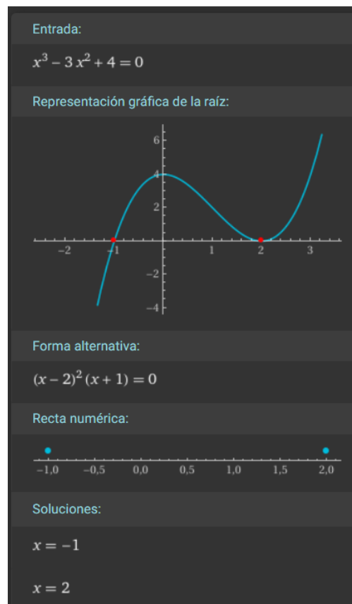
Figura 6: Comprobación matemática de la función cúbica en Wolfram Alpha.
